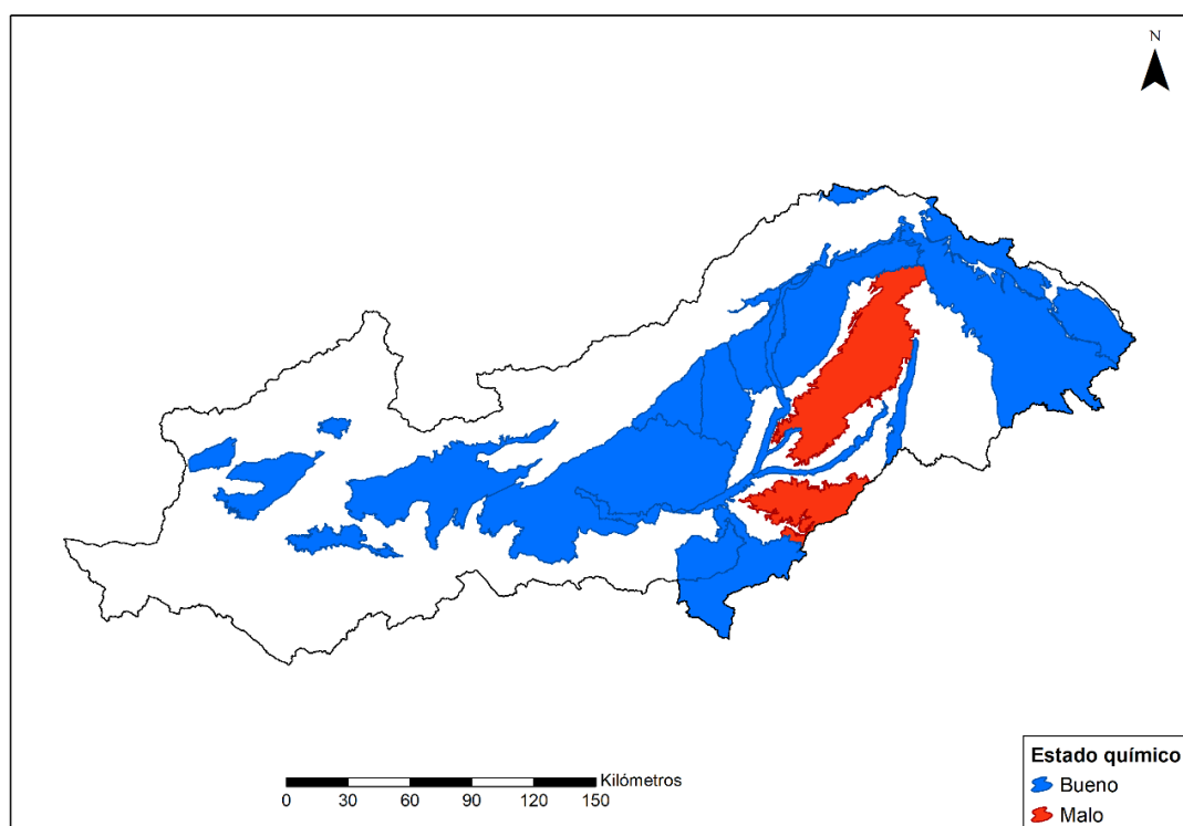
Figura 3. Estado químico (tercer ciclo de planificación) de las masas de agua subterránea de la parte española de la Demarcación Hidrográfica del Tajo
