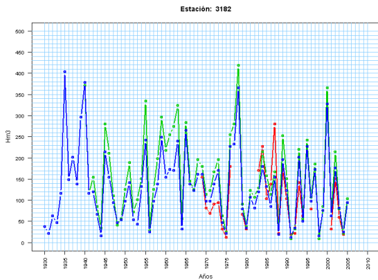
Figura 9. Serie aforada en cabecera del río Alagón
