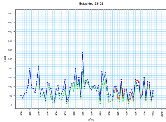
Figura 4. Serie de entradas en el embalse de Alcorlo en el río Bornova
