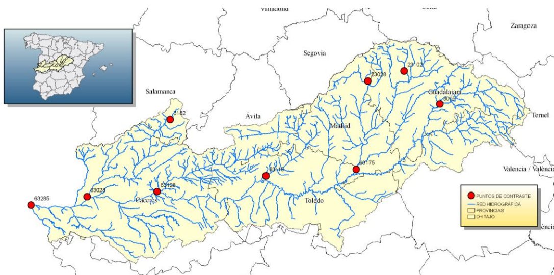
Figura 2. Mapa con la selección de puntos de control para la calibración del modelo
