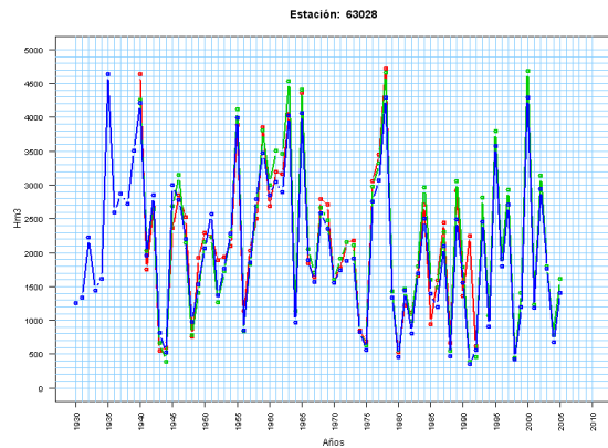
Figura 10. Serie restituida del Alagón completo
