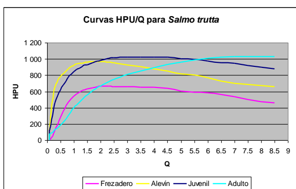
Figura 4. Ejemplo Curvas HPU/Q para un río modelo
