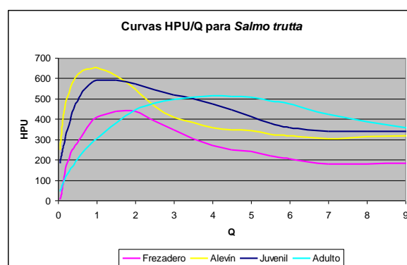
Figura 5. Ejemplo Curvas HPU/Q para otro cauce modelo
