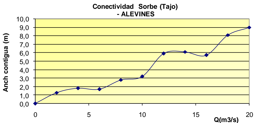
Figura 9. Gráfica de anchura de paso caudal par tramo unidimensional
