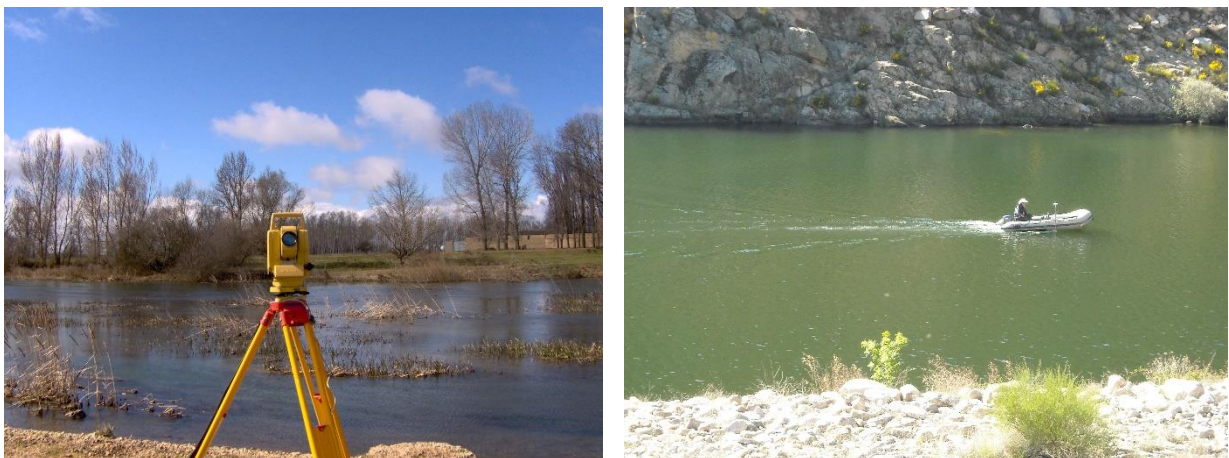
Figura 2. Toma de datos cauce mediante estación total y ecosonda acoplada a embarcación
