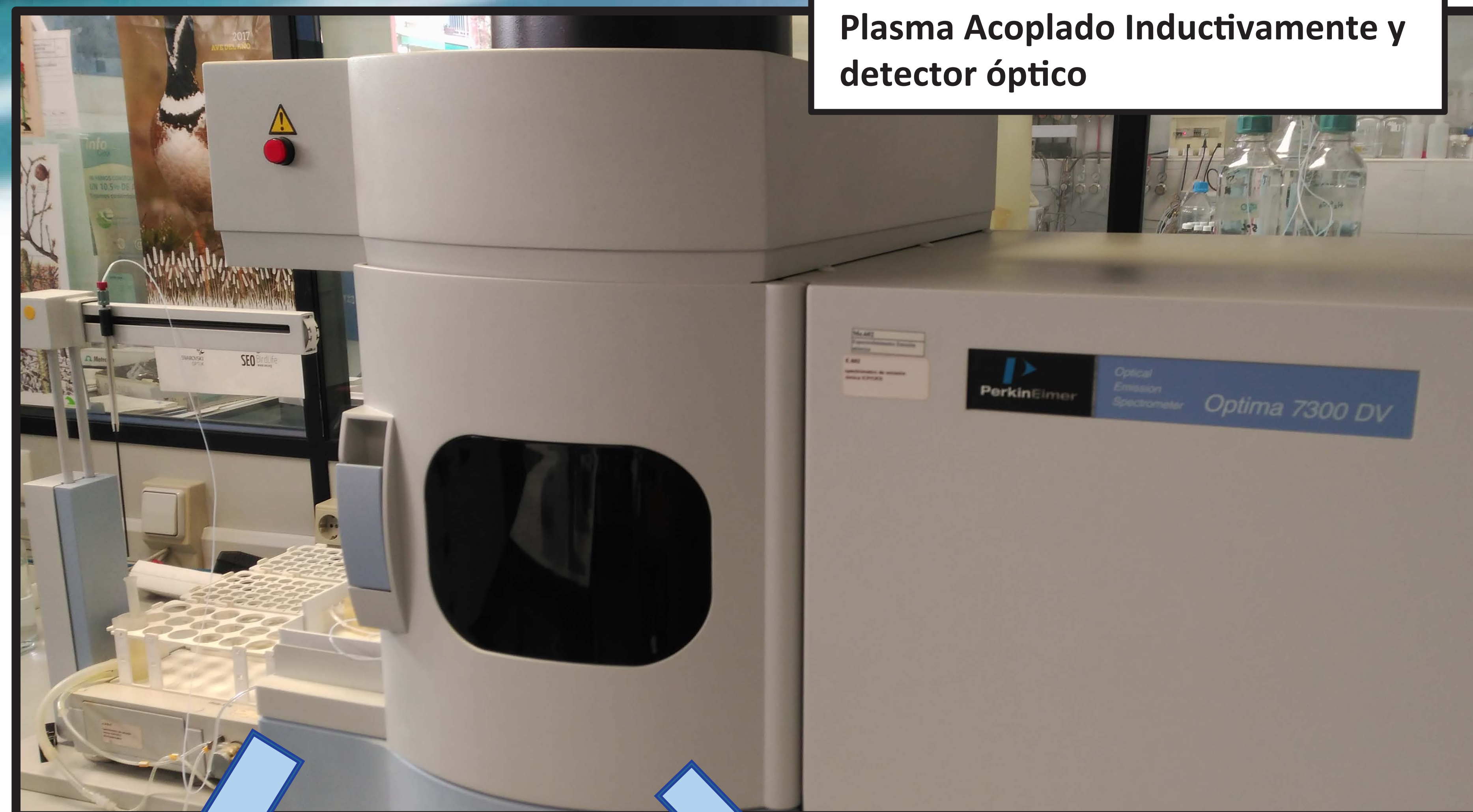
ICP-OES
