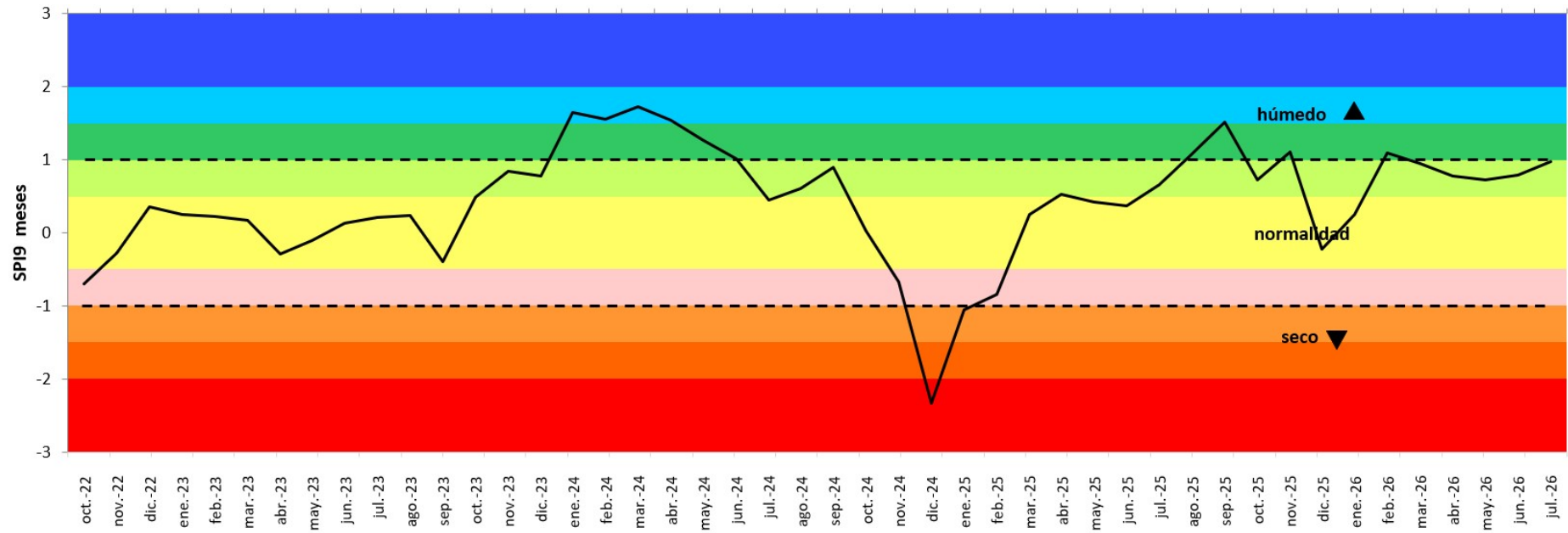
Índice Normalizado de Precipitación de los últimos 9 meses para la subcuenca del río Tago en España
