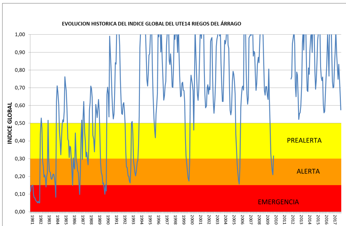
Figura 120. Evolución histórica del índice global de escasez de la UTE 14 Riegos del Árrago
