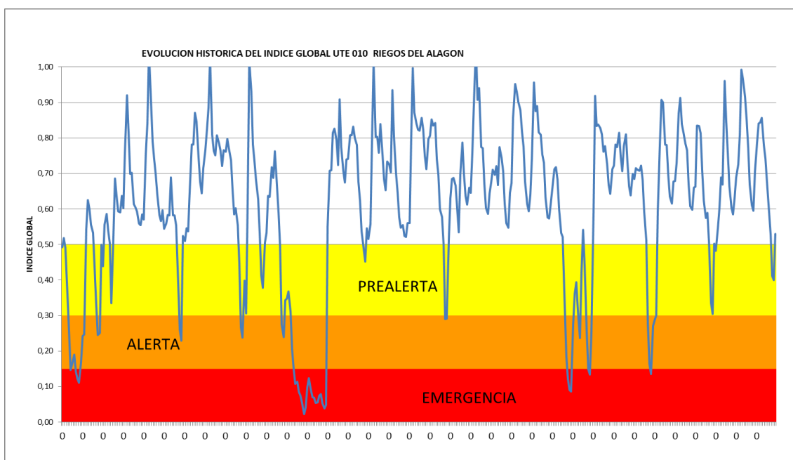
Figura 107. Evolución histórica del índice global de escasez de la UTE 10 Riegos del Alagón
