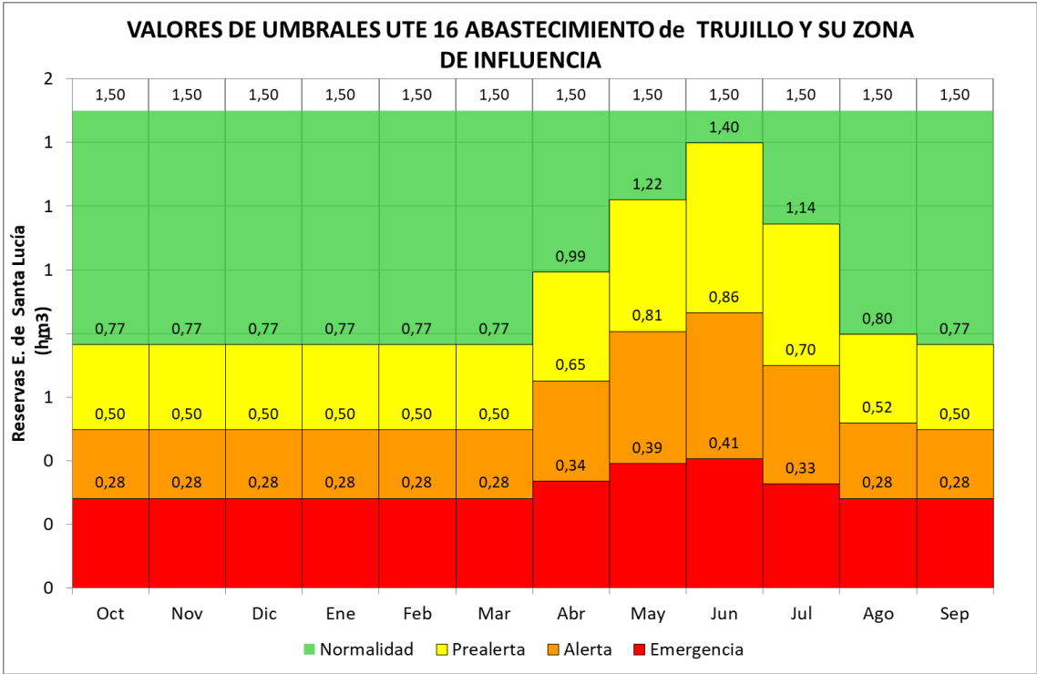
Figura 127. Umbrales de escasez UTE 17 Abastecimiento a Trujillo
