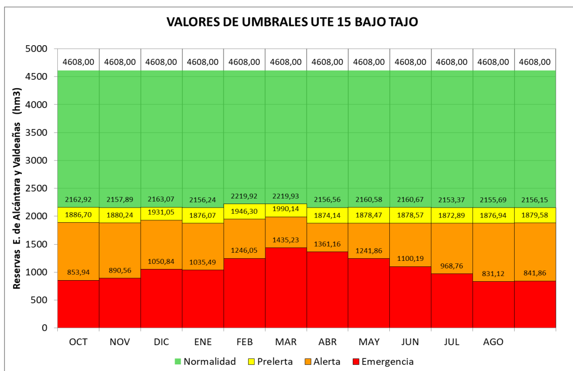
Figura 121. Umbrales de escasez UTE 15 Bajo Tajo – Extremadura
