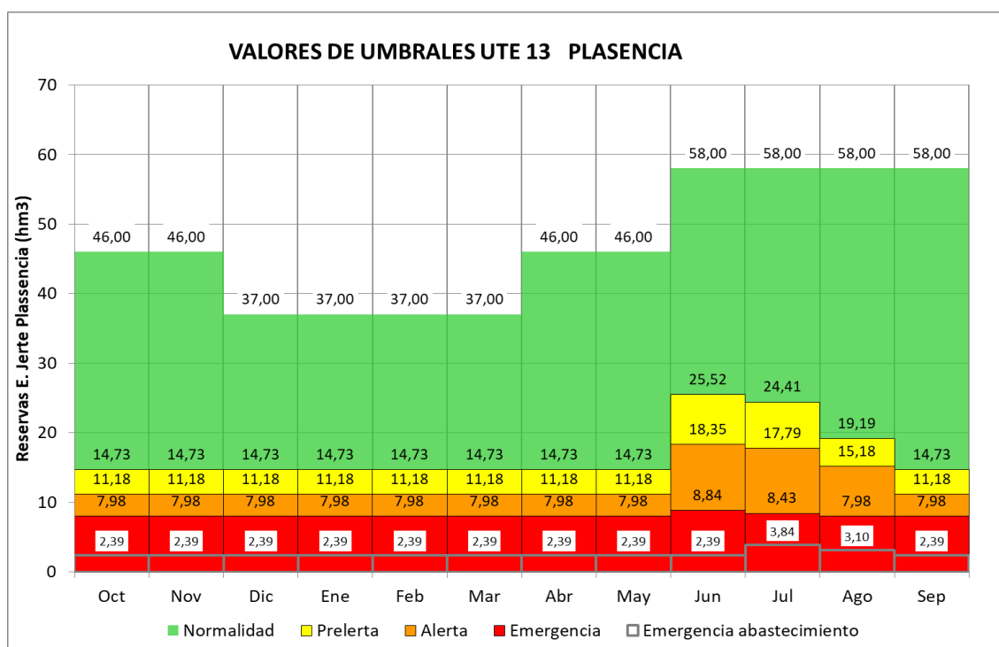
Figura 115. Umbrales de Escasez UTE 13 Abastecimiento a Plasencia
