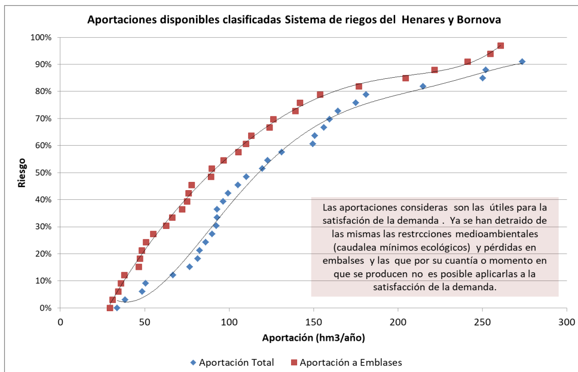
Figura 73. Aportaciones anuales disponibles clasificadas en la UTE 02 Riegos Tajuña
