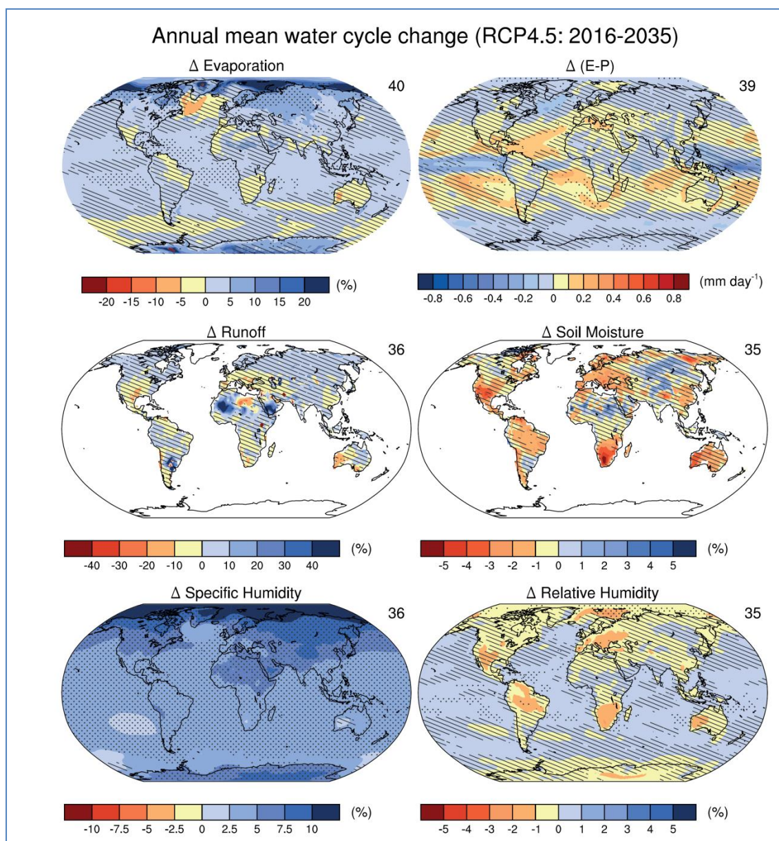
Figura 48. Proyección de cambios para el periodo 2016-2031 para: evaporación (%), evaporación menos precipitación (mm/día), escorrentía total (%), humedad del suelo en los 10 cm superiores (%), cambio relativo en humedad específica (%) y cambio absoluto en humedad relativa (%). El número en la parte superior derecha de la imagen indica el número de modelos promediados. Fuente: Kirtman y otros (2013).
