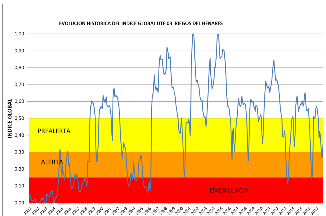
Figura 76. Evolución histórica del índice global de la UTE 03 Riegos del Henares
