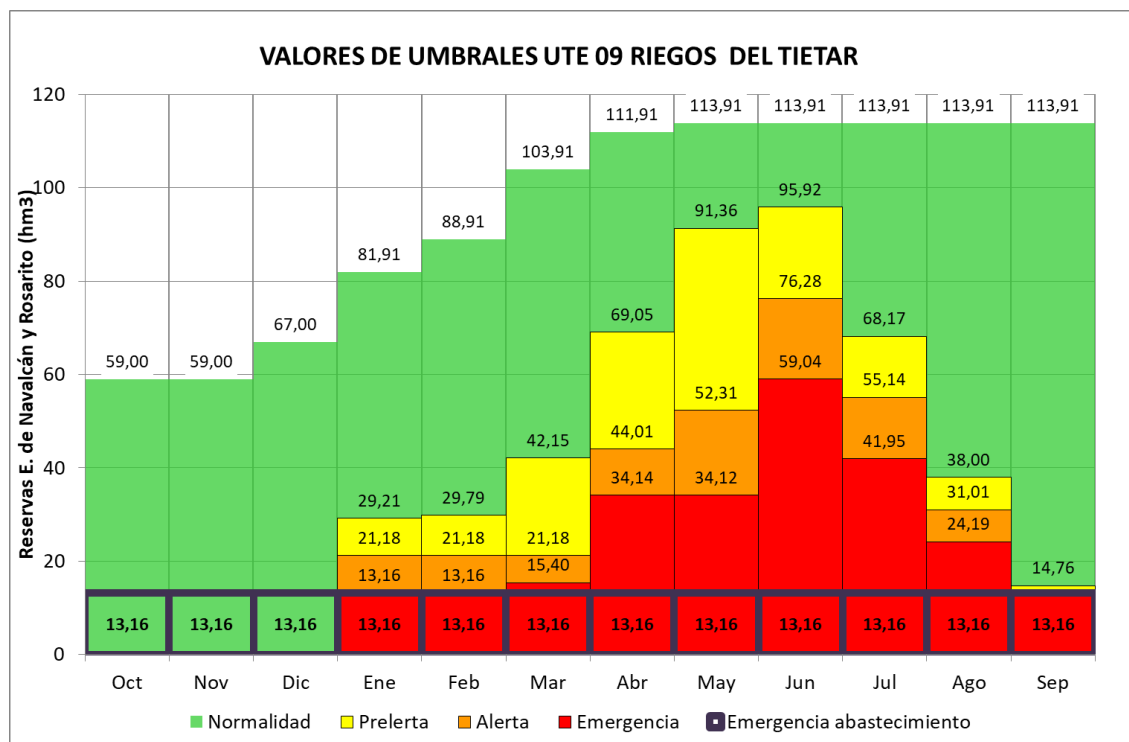
Figura 102. Umbrales de escasez UTE 09 Riegos del Tiétar
