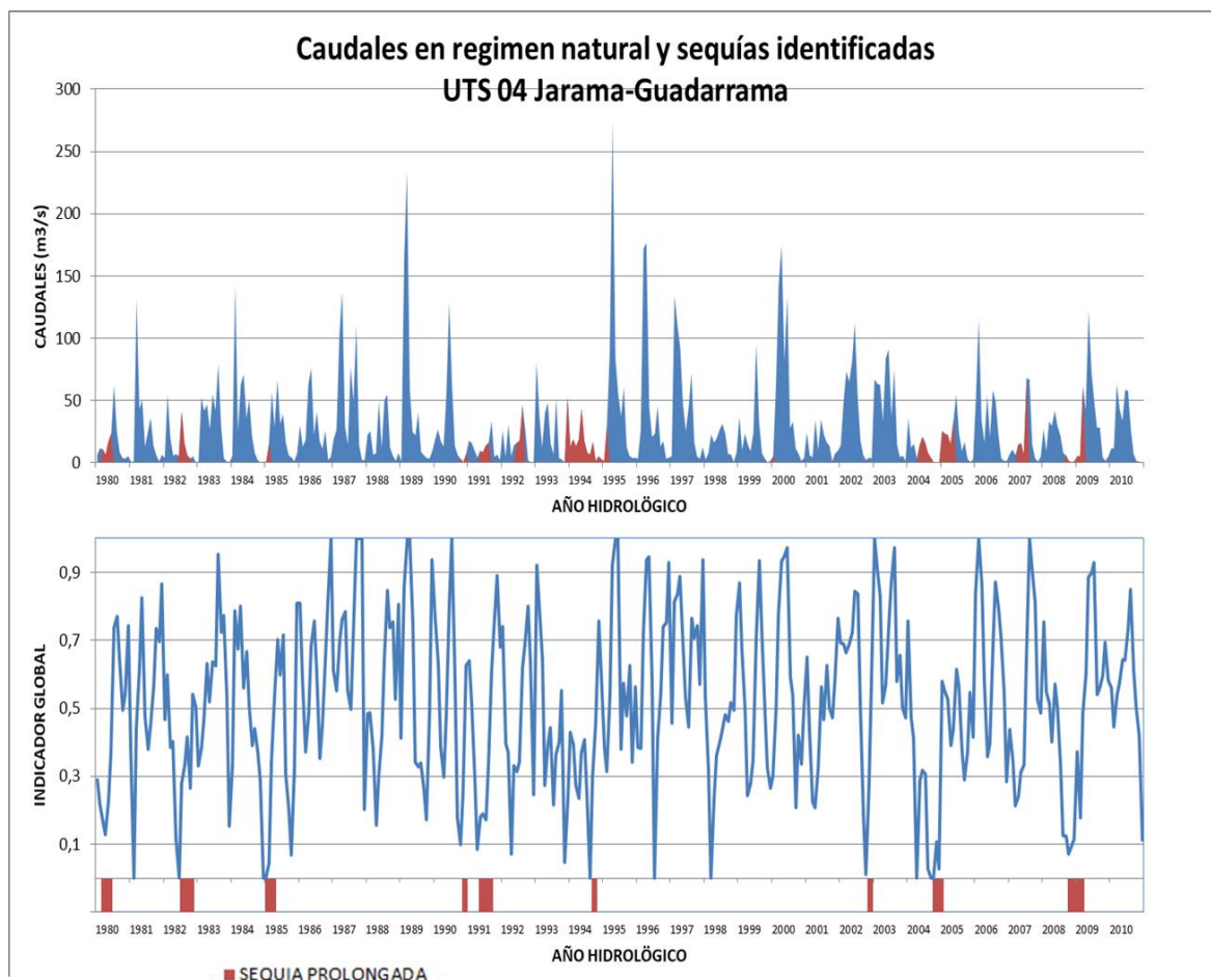
Figura 60. Caudales en régimen natural y sequías identificadas en la UTS 04 Jarama - Guadarrama
