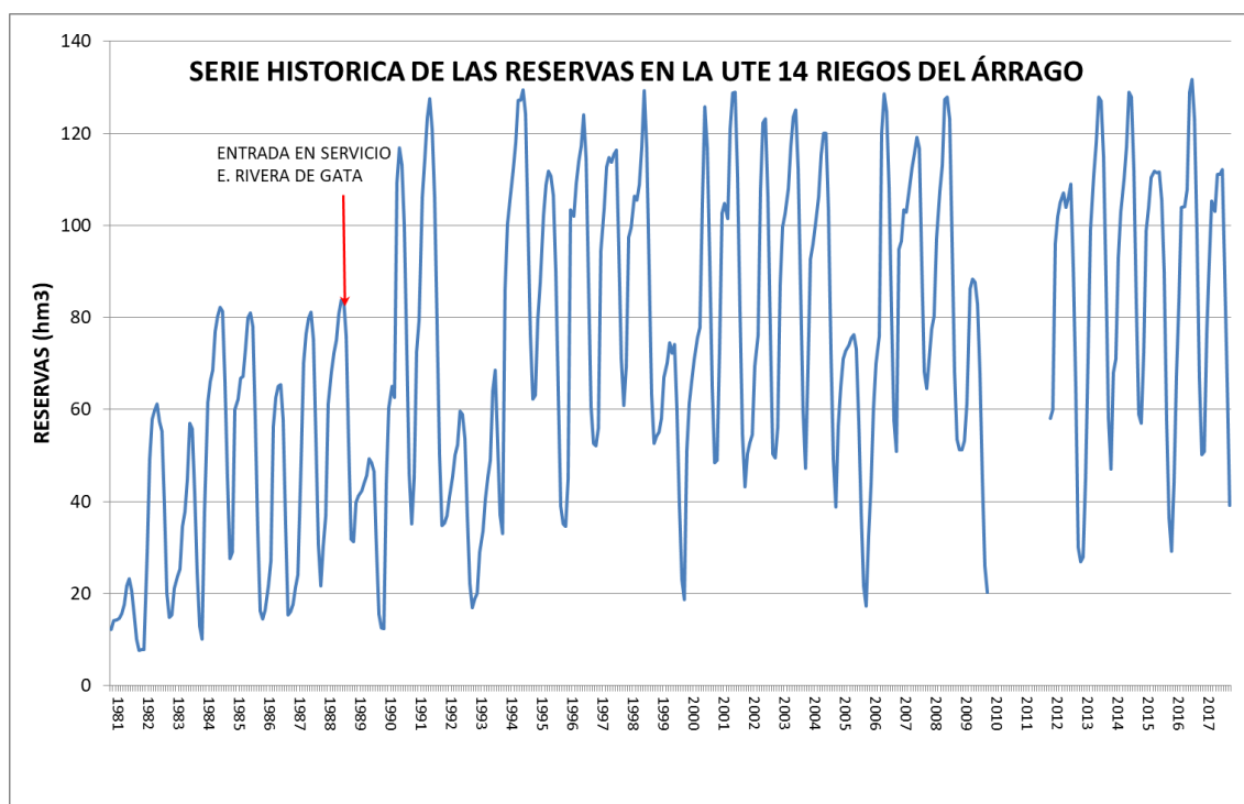
Figura 119. Evolución histórica del indicador de escasez de la UTE 14 Riegos del Árrago
