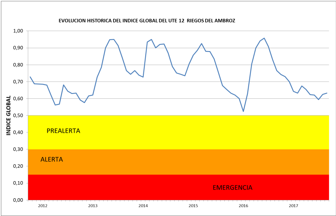
Figura 114. Evolución histórica del índice global de escasez de la UTE 12 Riegos del Ambroz
