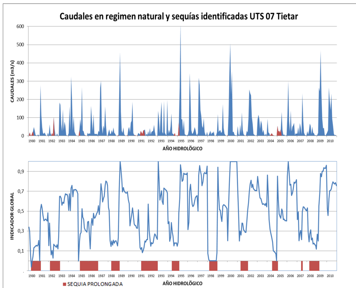
Figura 63. Caudales en régimen natural y sequías identificadas en la UTS 07 Tiétar
