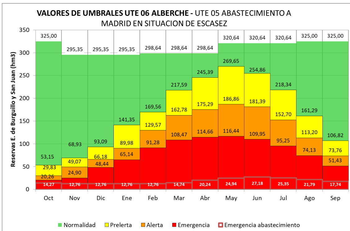
Figura 89. Umbrales UTE 06 para UTE 05 Abastecimiento a Madrid en Escasez
