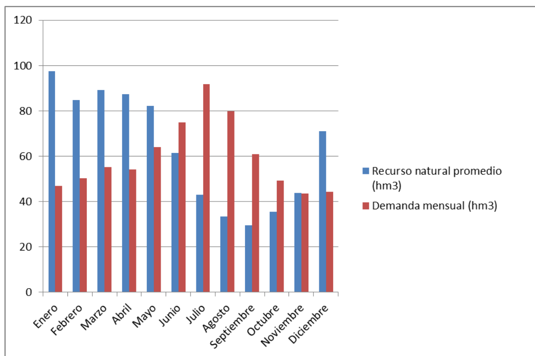
Figura 9. Curvas de demanda y recurso en régimen natural mensual para año tipo en la UTE 01 Trasvase ATS
