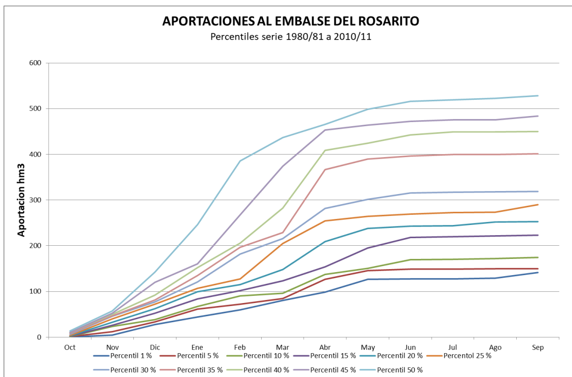
Figura 99. Percentiles de aportaciones al embalse de Rosarito
