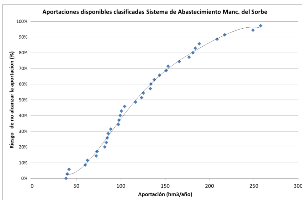
Figura 77. Aportaciones probables E. Beleña UTE 04 Abastecimiento Mancomunidad de Aguas del Sorbe
