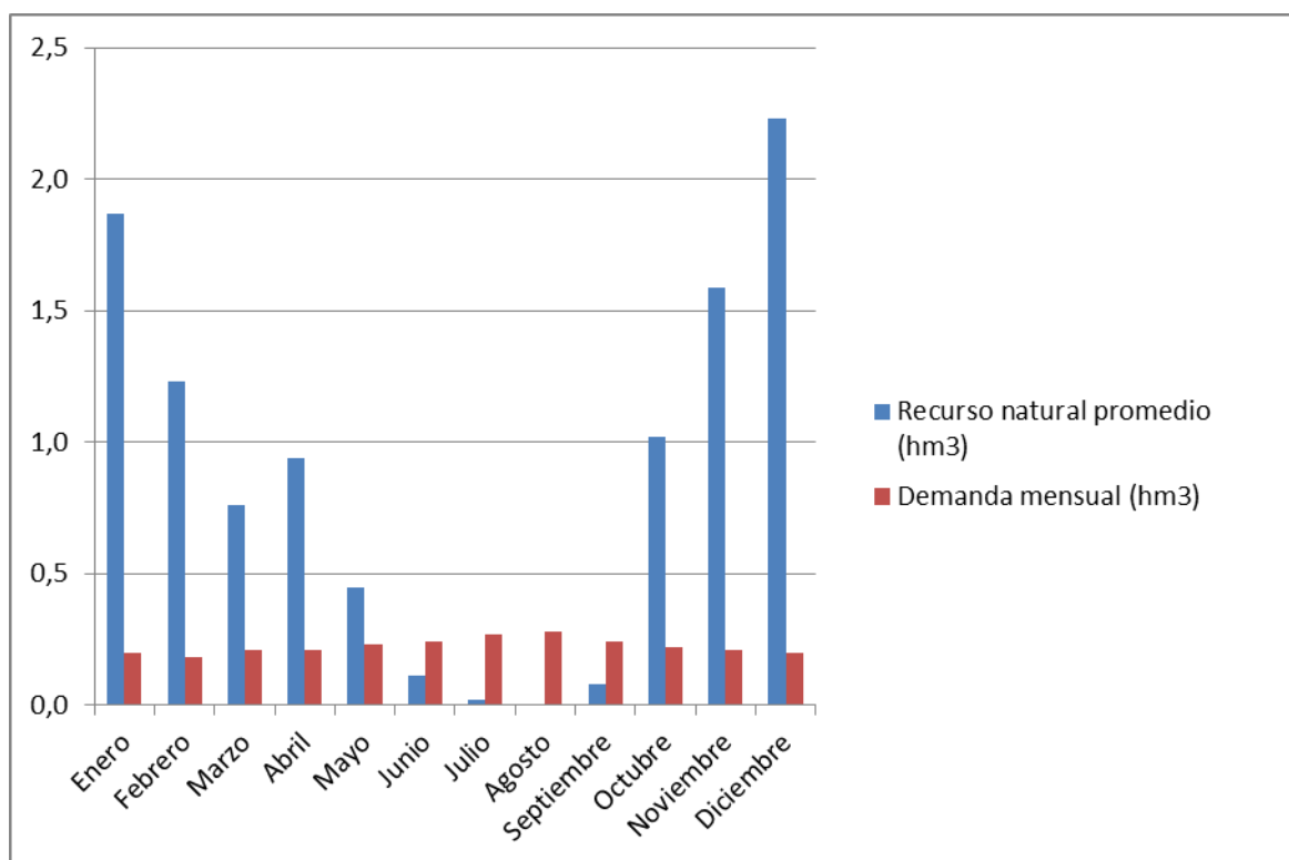
Figura 45. Curvas de demanda y recurso en régimen natural mensual para año tipo en la UTE 17 Abastecimiento a Trujillo
