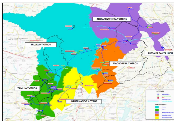
Figura 43. Esquema de funcionamiento de la UTE 17 Abastecimiento a Trujillo
