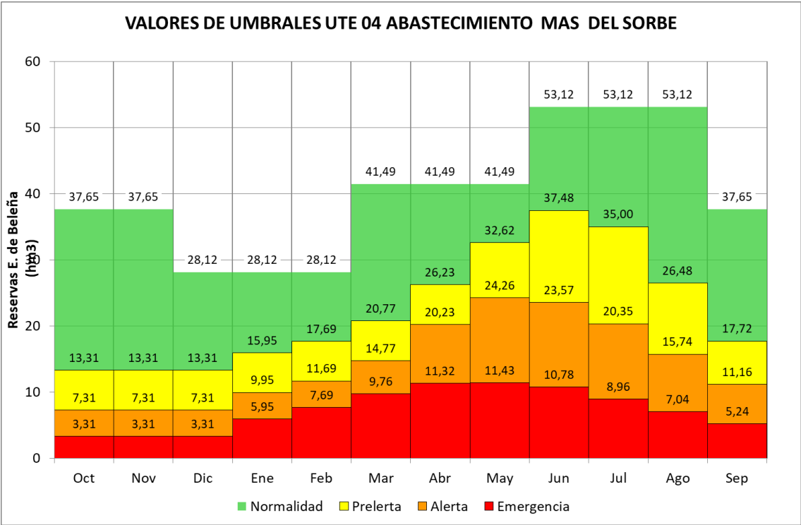
Figura 78. Umbrales mensuales de Escasez UTE 04 MAS del Sorbe
