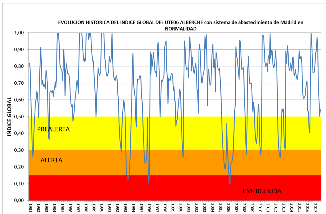
Figura 91. Evolución histórica del índice global de escasez de la UTE 06 Alberche. UTE 05 Abastecimiento a Madrid en Normalidad
