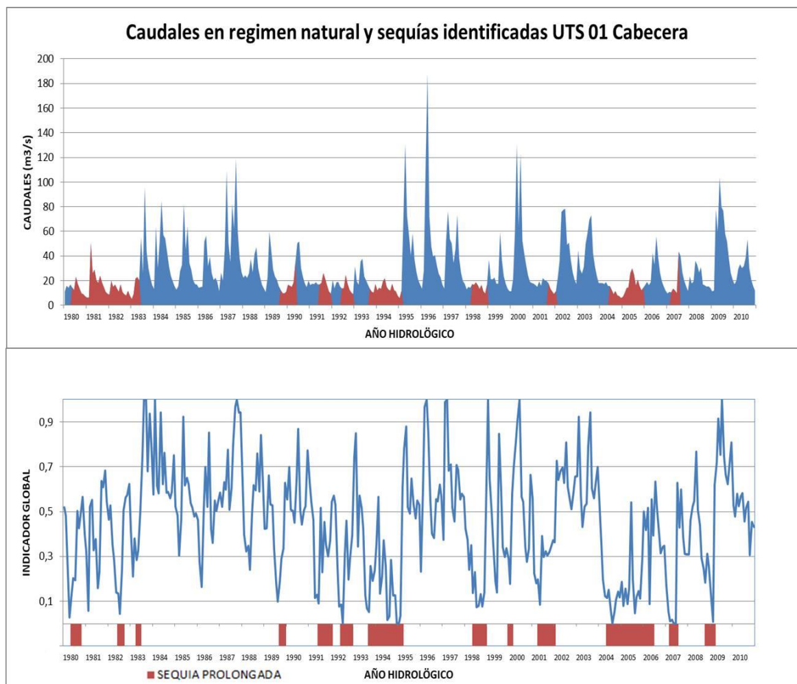
Figura 57. Caudales en régimen natural y sequías identificadas en la UTS 01 Cabecera
