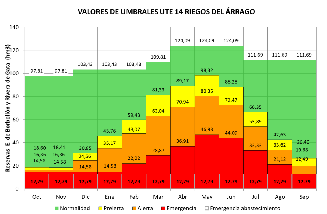
Figura 118. Umbrales de escasez UTE 14 Riegos del Árrago
