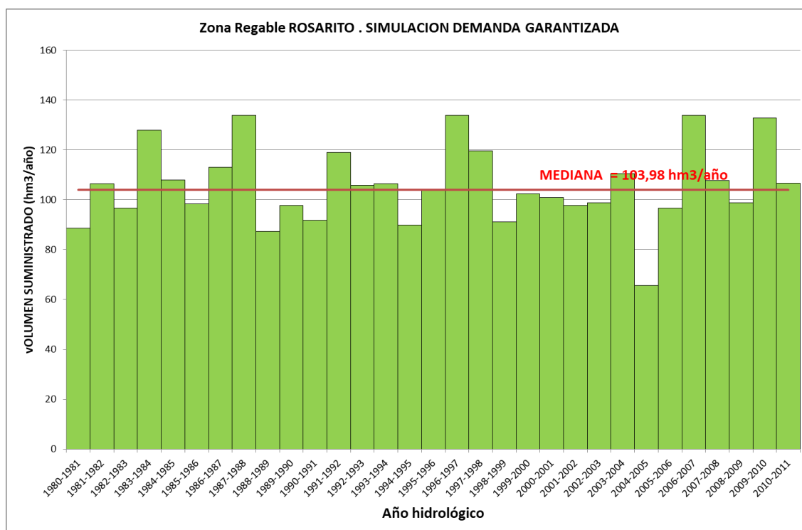
Figura 100. Demandas garantizadas (simulación) Zona Regable Rosarito
