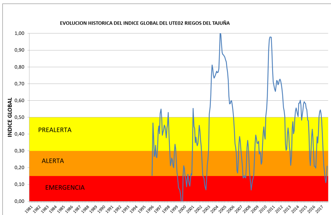
Figura 72. Evolución histórica del índice global de escasez de la UTE 02 Riegos del Tajuña
