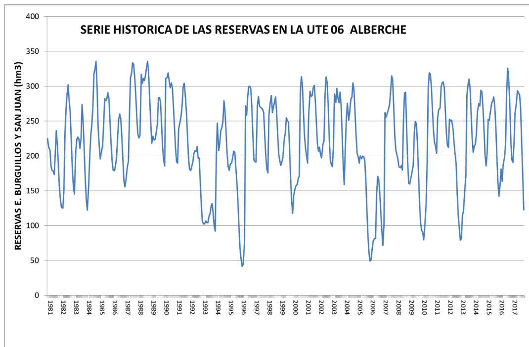
Figura 90. Evolución histórica del indicador de escasez de la UTE 06 Alberche
