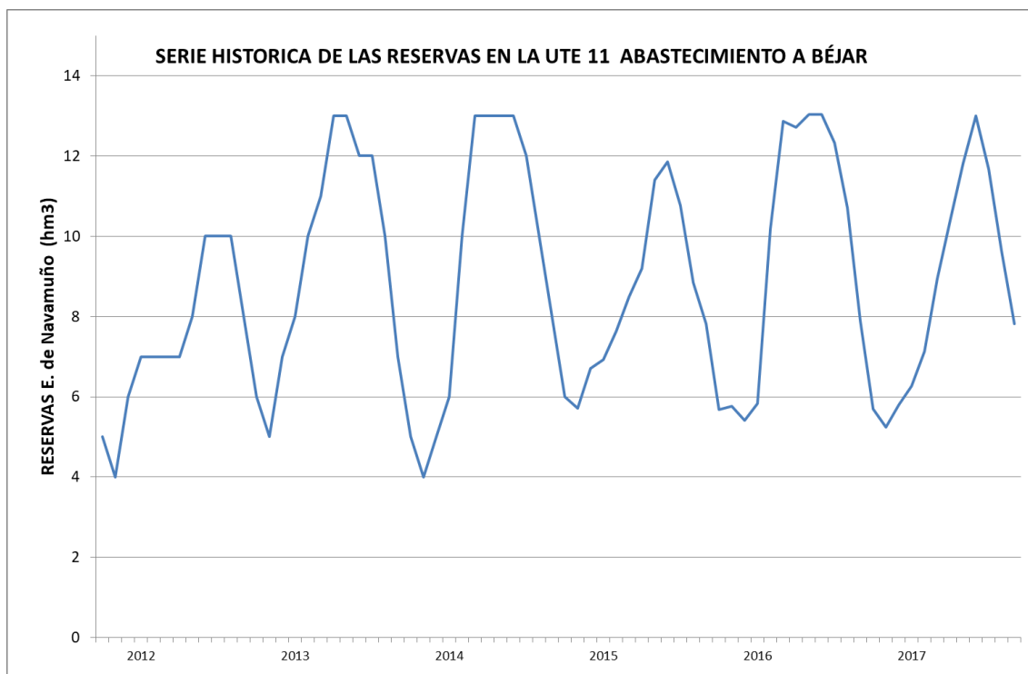
Figura 110. Evolución 2011/12 A 2016/17 del indicador de escasez de la UTE 11 Abastecimiento a Béjar y su zona de influencia
