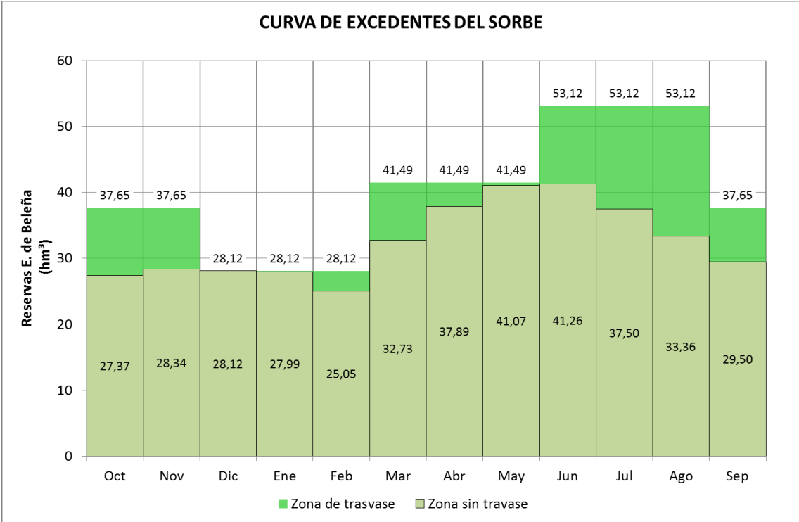
Figura 83. Curva de derivación del Azud Pozo de los Ramos al canal del Jarama
