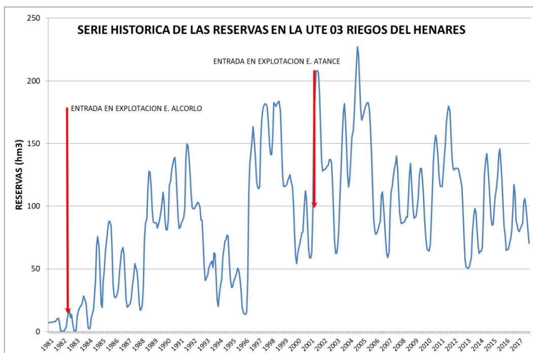
Figura 75. Evolución histórica del indicador de escasez de la UTE 03 Riegos del Henares
