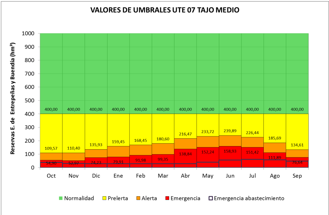
Figura 93. Umbrales UTE 07 Tajo Medio
