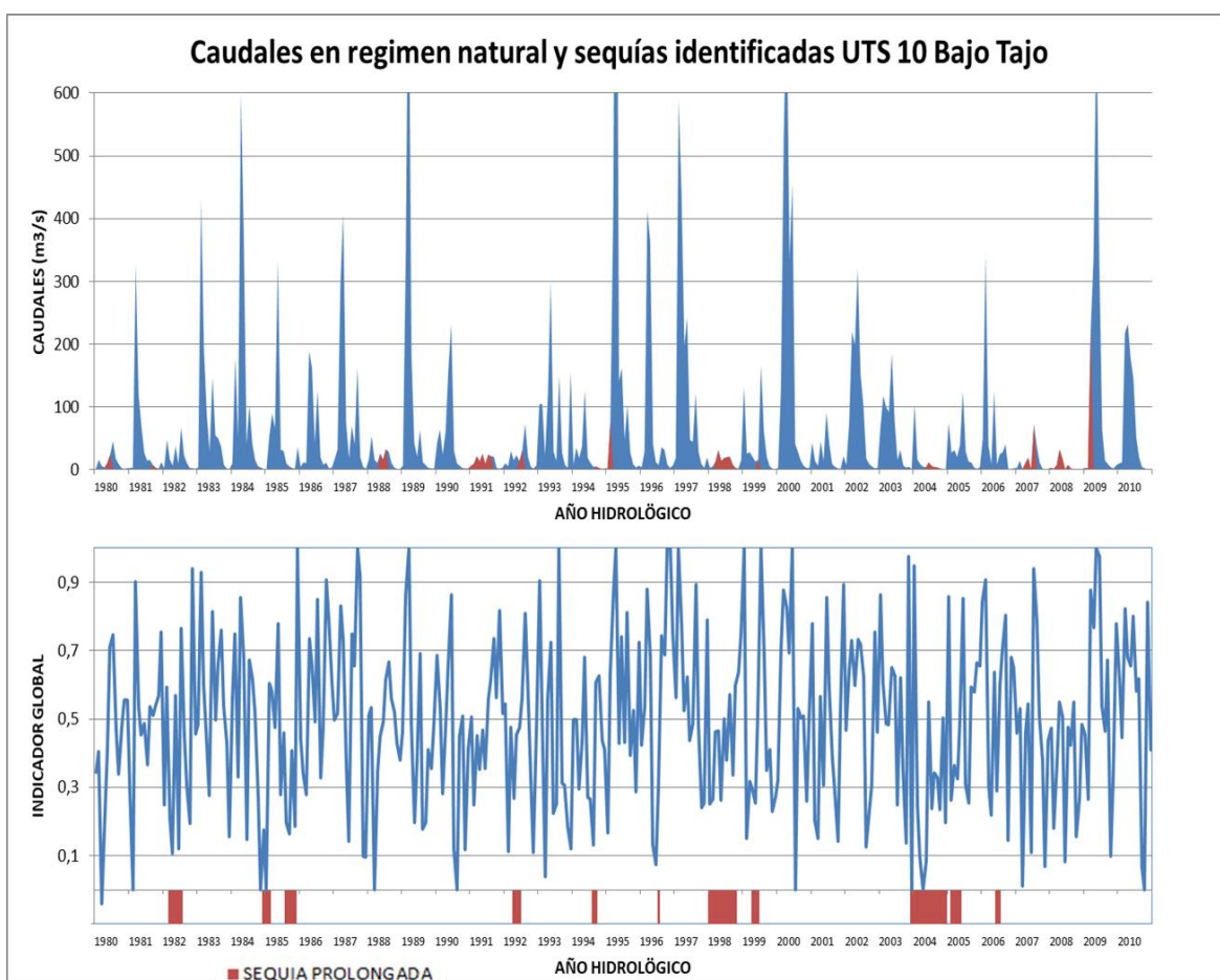
Figura 66. Caudales en régimen natural y sequías identificadas en la UTS 10 Bajo Tajo
