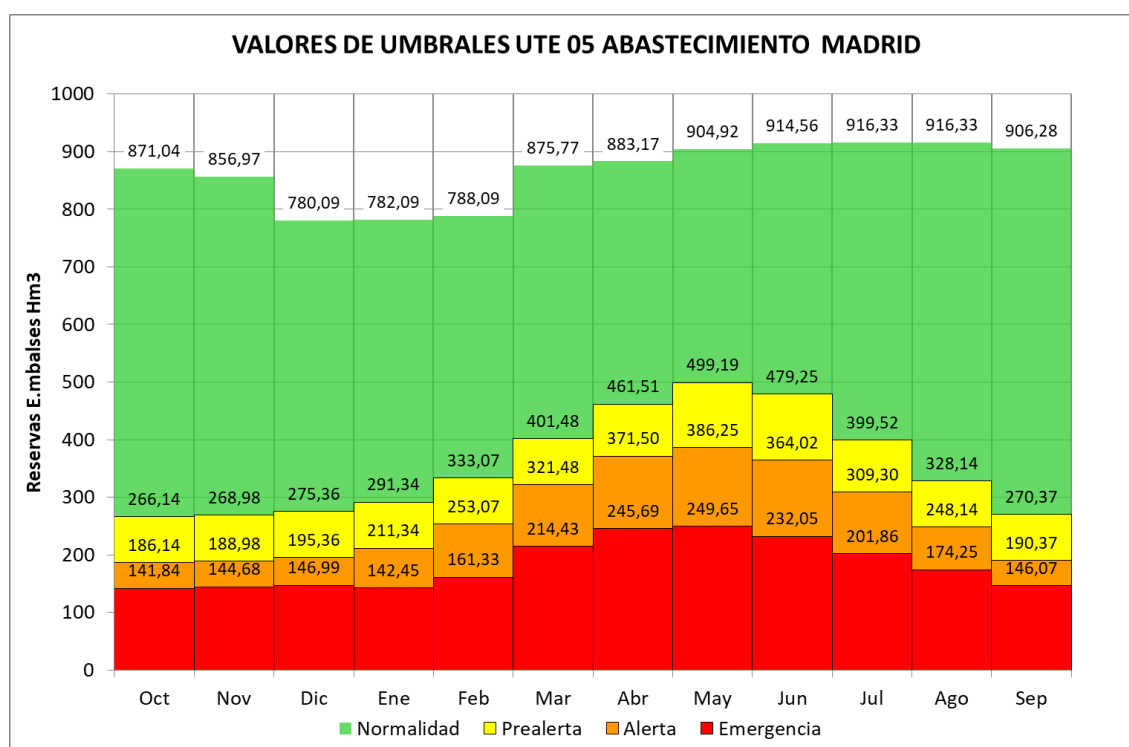
Figura 84. Umbrales de Escasez UTE 05 Abastecimiento de Madrid
