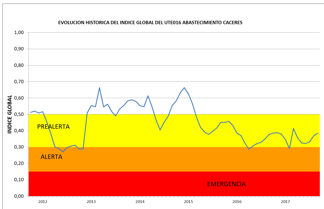
Figura 125. Evolución histórica índice global de escasez de escasez UTE 16 Abastecimiento a Cáceres
