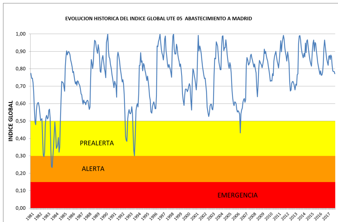
Figura 87. Evolución histórica del índice global de escasez de la UTE 05 Abastecimiento de Madrid
