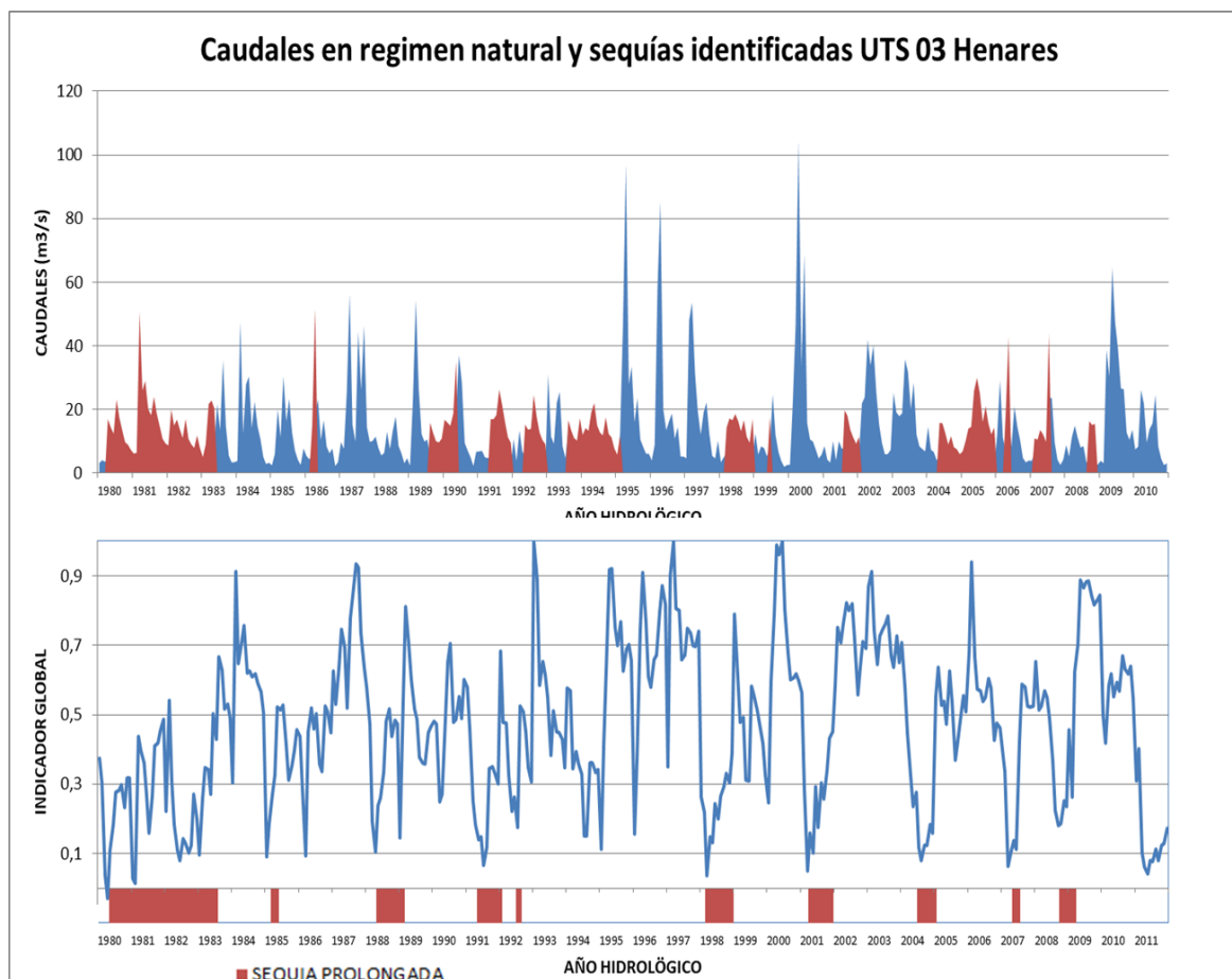
Figura 59. Caudales en régimen natural y sequías identificadas en la UTS 03 Henares
