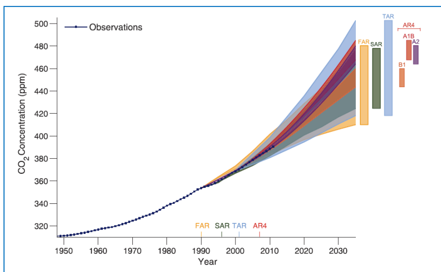
Figura 47. Evolución de las emisiones de CO 2 previstas por distintos escenarios y datos observados. Fuente: Cubasch y otros (2013).
