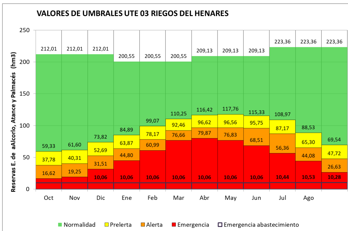
Figura 74. Umbrales de Escasez UTE 03 Riegos del Henares
