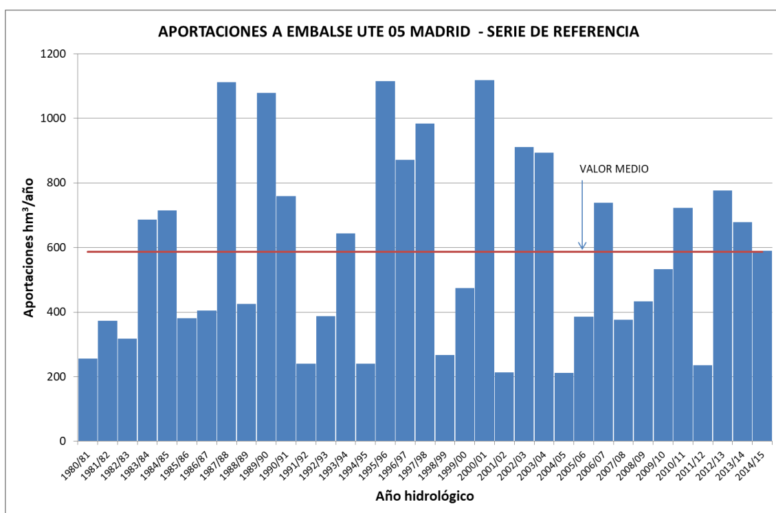
Figura 82. Aportaciones anuales UTE 05 Abastecimiento Madrid
