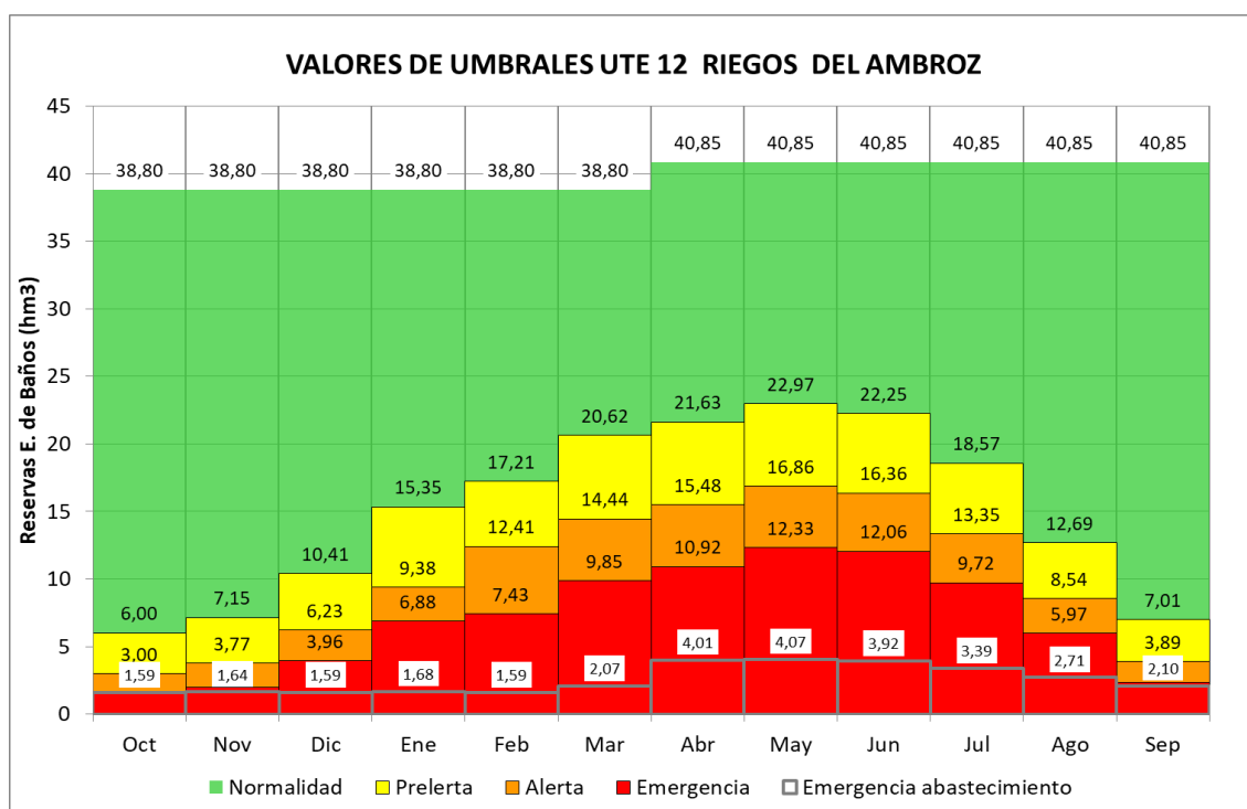
Figura 112. Umbral de Escasez UTE 12 Riegos del Ambroz
