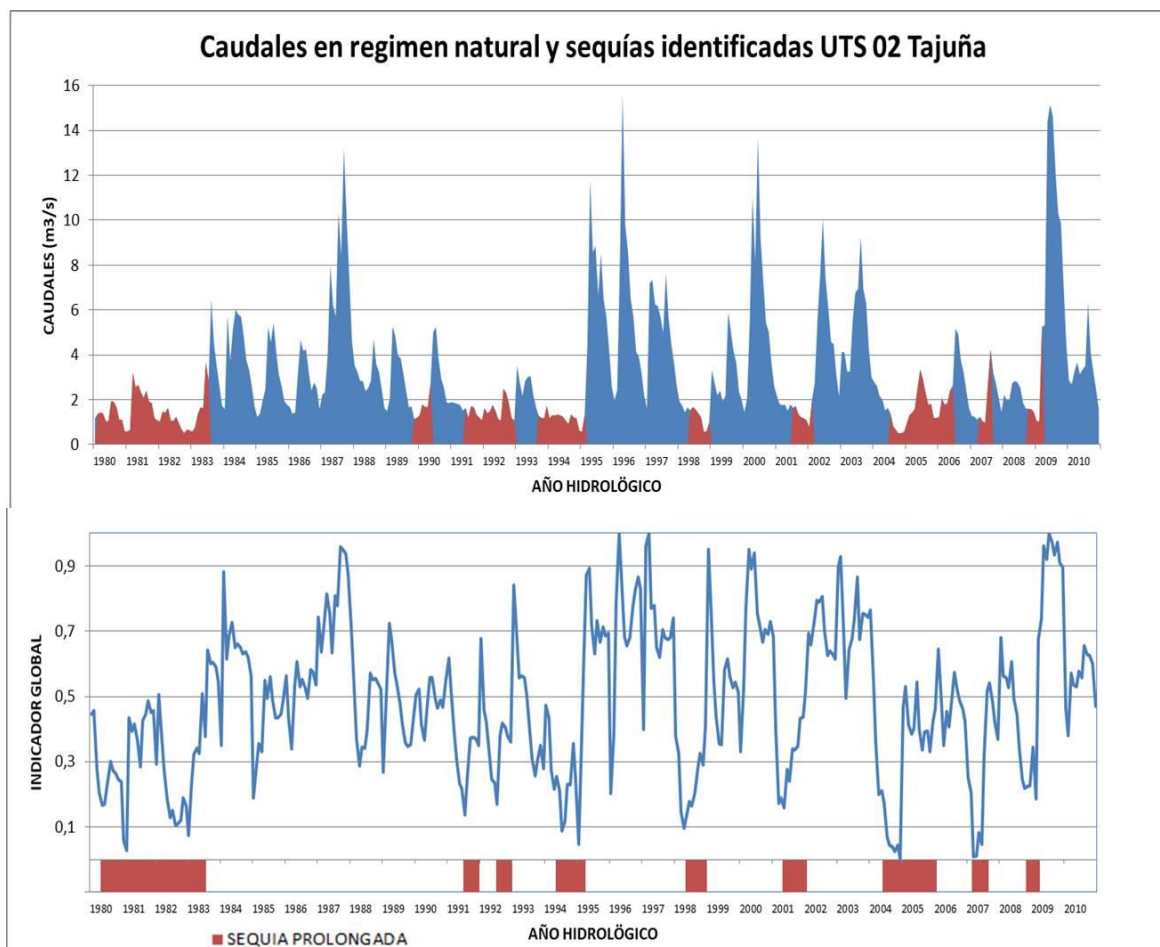
Figura 58. Caudales en régimen natural y sequías identificadas en la UTS 02 Tajuña
