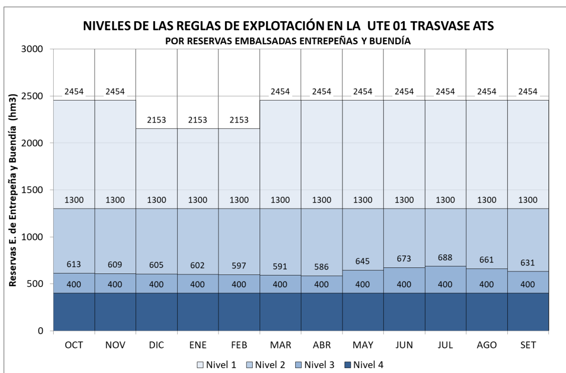
Figura 69. Niveles de las reglas de explotación en la UTE 01 Traslase ATS, por reservas embalsadas en Entrepeñas y Buendía
