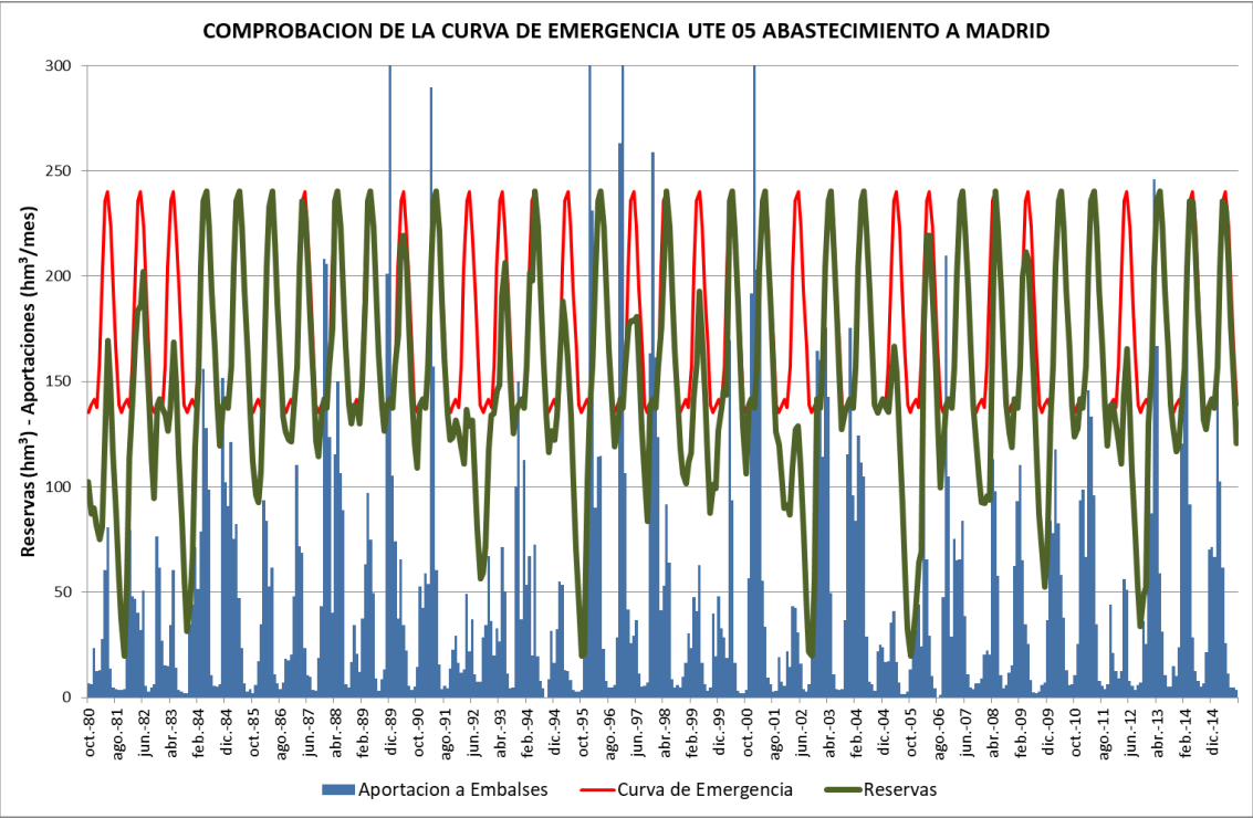
Figura 85. Comprobación del Umbrales de Emergencia UTE 05 Abastecimiento de Madrid
