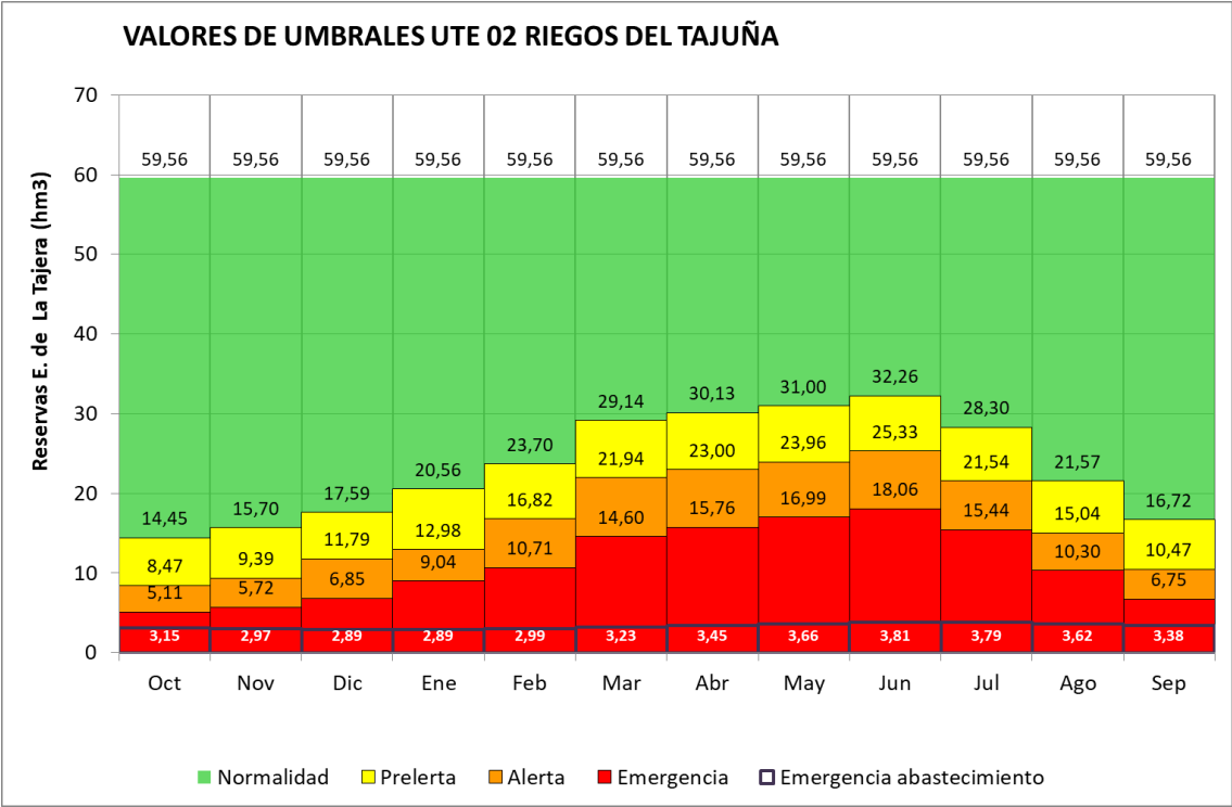
Figura 70. Umbrales de Escasez UTE 02 Riegos Tajuña
