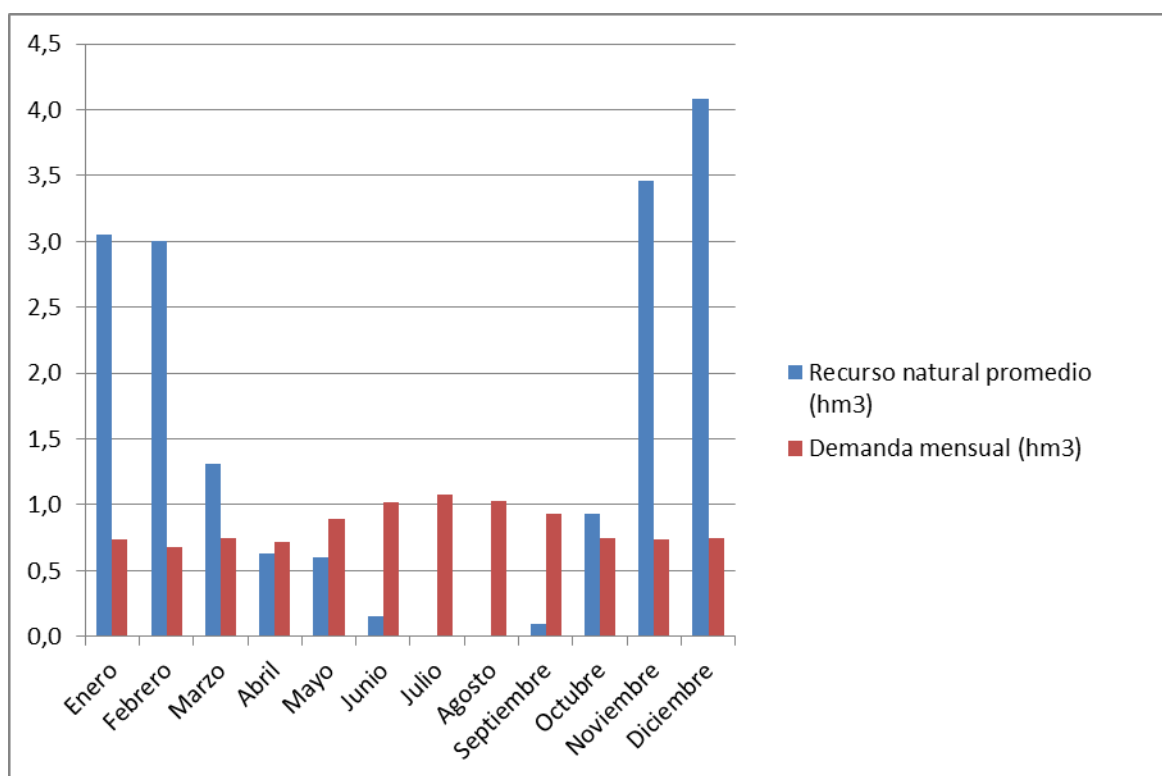
Figura 42. Curvas de demanda y recurso en régimen natural mensual para año tipo en la UTE 16 Abastecimiento a Cáceres
