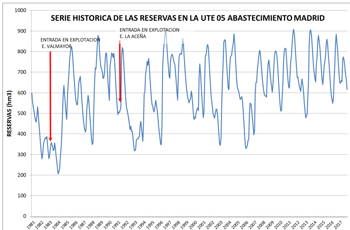
Figura 86. Evolución histórica del indicador de escasez de la UTE 05 Abastecimiento de Madrid
