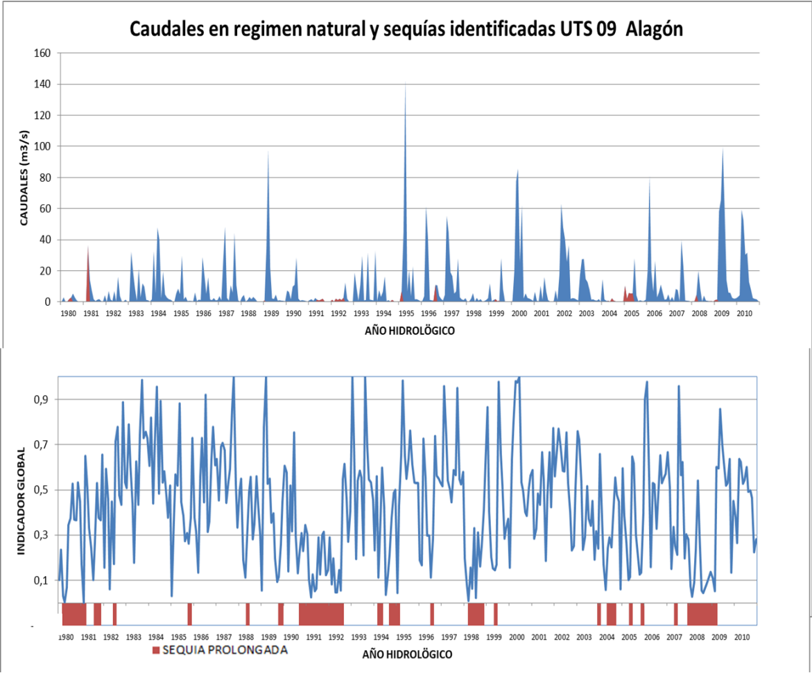
Figura 65. Caudales en régimen natural y sequías identificadas en la UTS 09 Alagón
