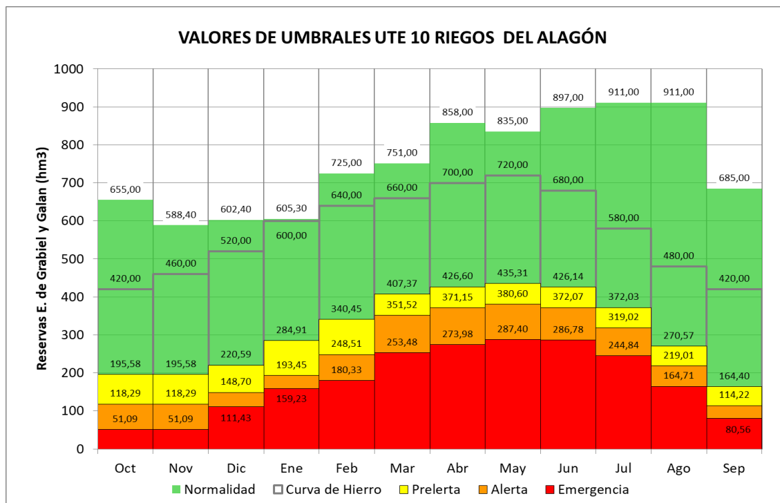
Figura 105. Umbrales de Escasez UTE 10 Riegos del Alagón
