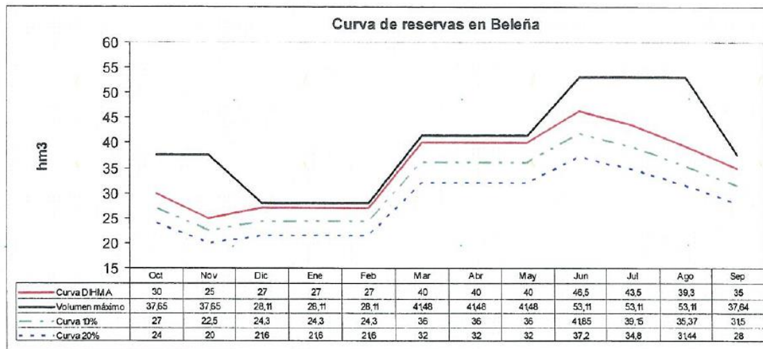
Figura 15. Curva antigua de excedentes en el Sorbe
