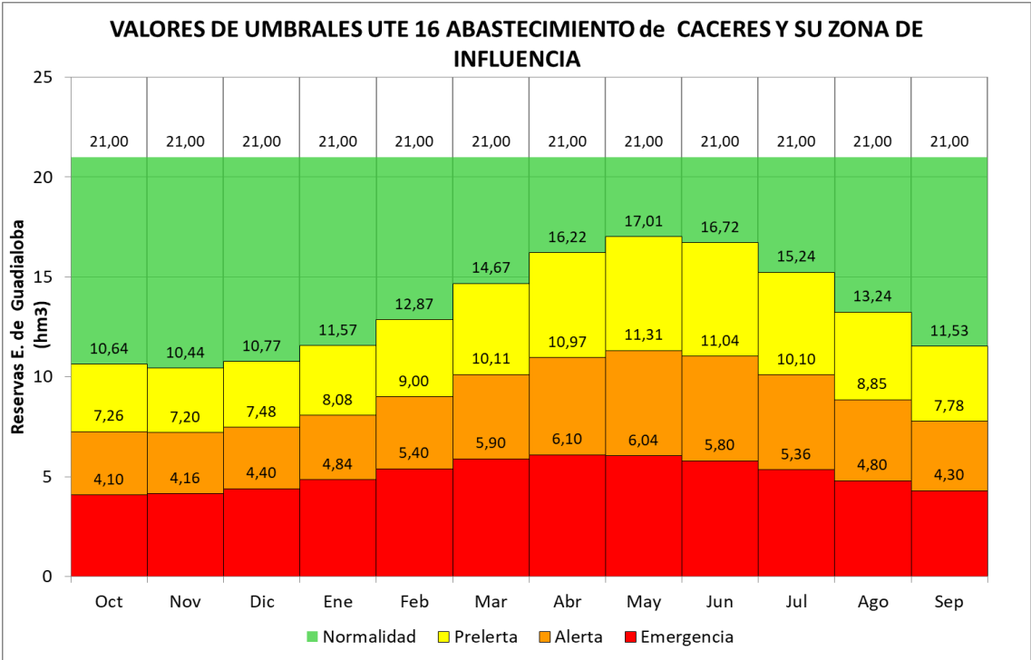
Figura 123. Umbral de escasez UTE 16 Abastecimiento a Cáceres
