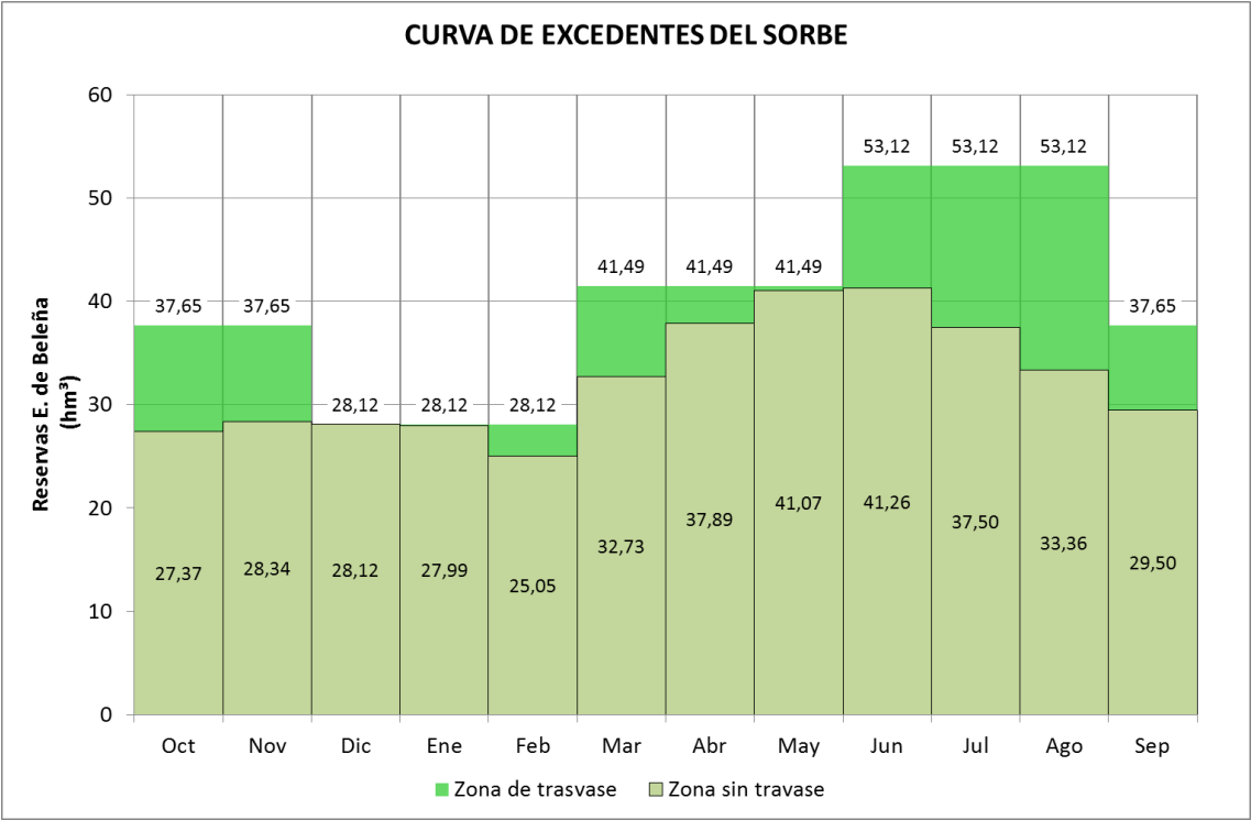
Figura 80. Curva de excedentes del Sorbe en el embalse de Beleña
