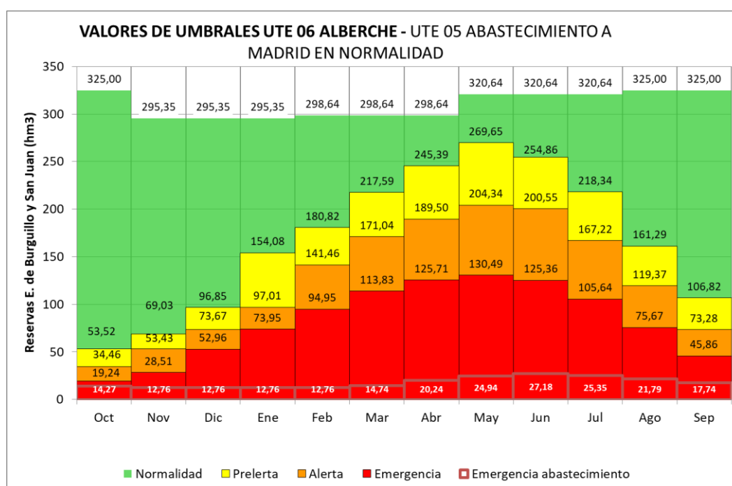
Figura 88. Umbrales UTE 06 para UTE 05 Abastecimiento a Madrid en Normalidad
