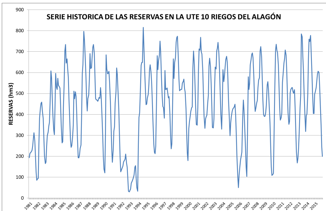
Figura 106. Evolución histórica del indicador de escasez de la UTE 10 Riegos del Alagón
