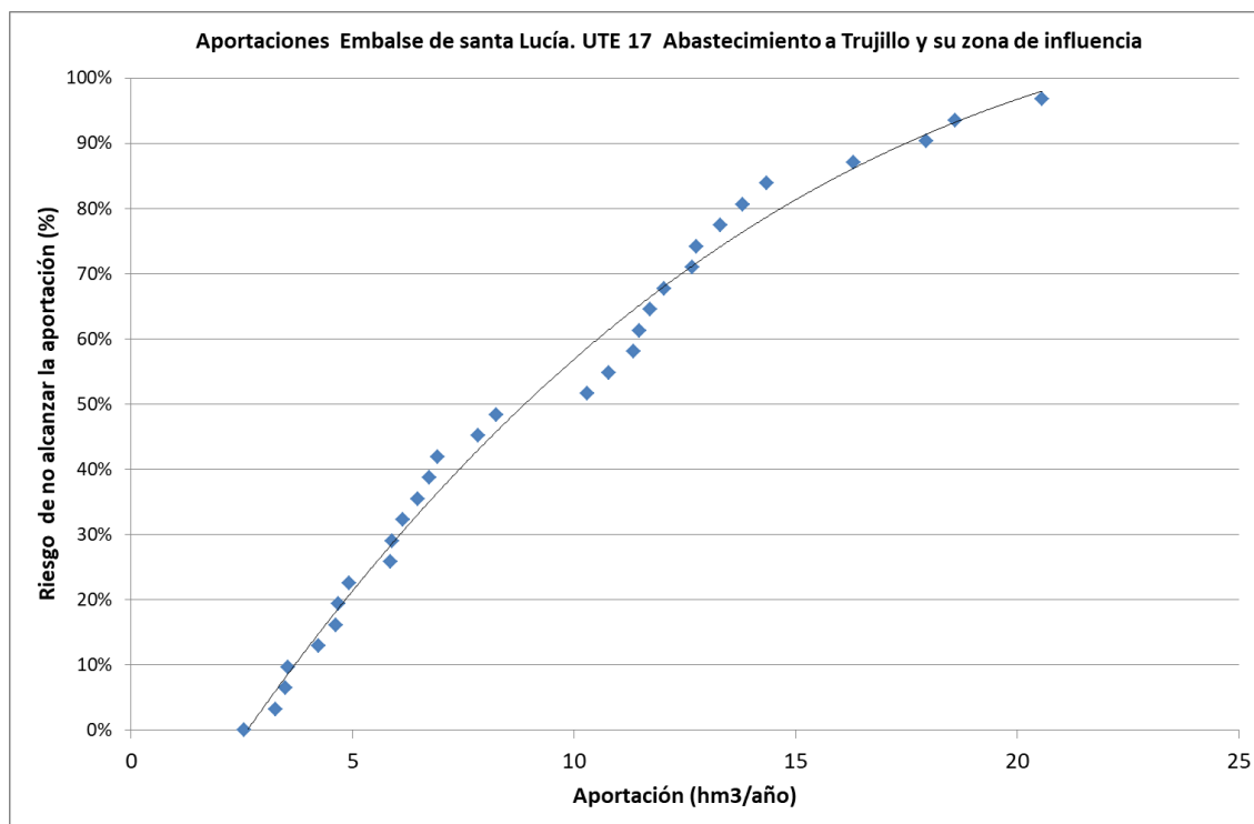
Figura 126. Aportaciones probables E. Guadiloba UTE 17 Abastecimiento a Trujillo
