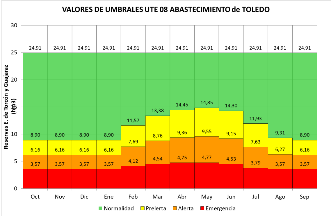
Figura 96. Umbrales de Escasez UTE 08 Abastecimiento a Toledo
