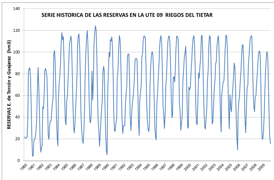
Figura 103. Evolución histórica del indicador de escasez de la UTE 09 Riegos del Tietar
