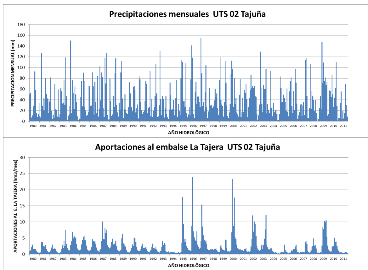
Figura 54. Evolución histórica de los registros de precipitaciones y aportaciones en UTS 02 Tajuña
