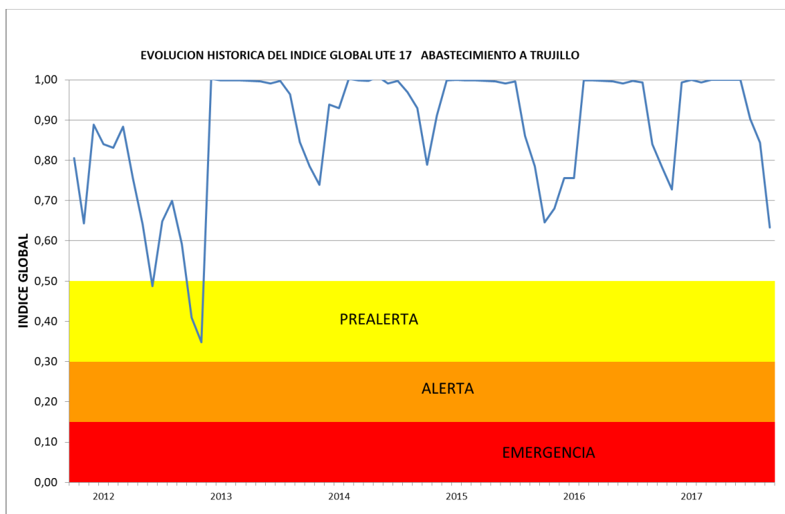
Figura 129. Evolución histórica del índice global de escasez de la UTE 17 Abastecimiento a Trujillo
