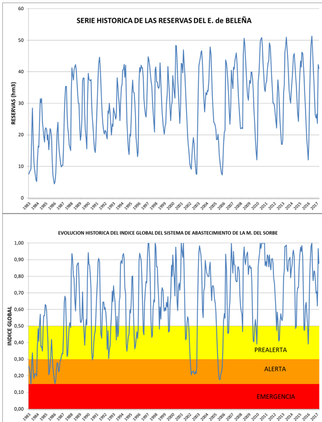
Figura 79. Evolución del Indicador de La UTE 04 MAS del Sorbe
