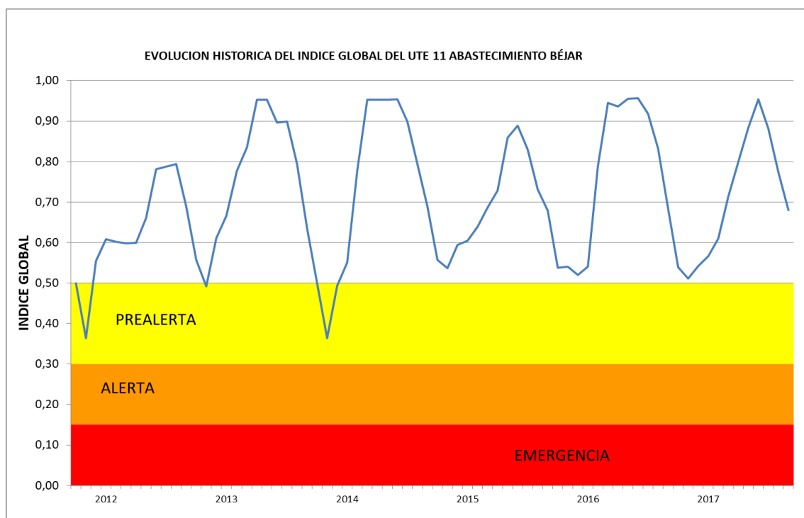
Figura 111. Evolución histórica del índice global de escasez de la UTE 11 abastecimiento a Béjar y su zona de influencia
