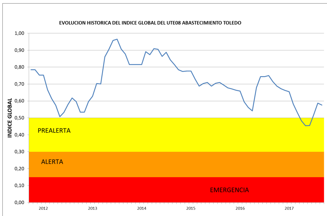
Figura 98. Evolución histórica del índice global de escasez de la UTE 08 abastecimiento a Toledo
