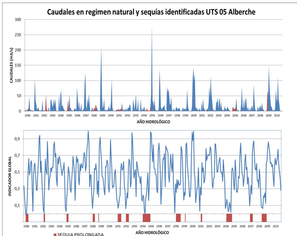
Figura 61. Caudales en régimen natural y sequías identificadas en la UTS 05 Alberche
