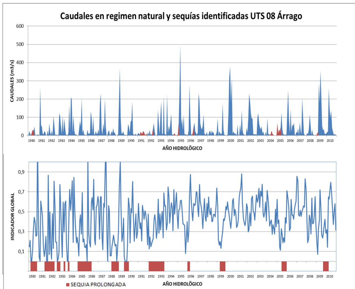
Figura 64. Caudales en régimen natural y sequías identificadas en la UTS 08 Árrago
