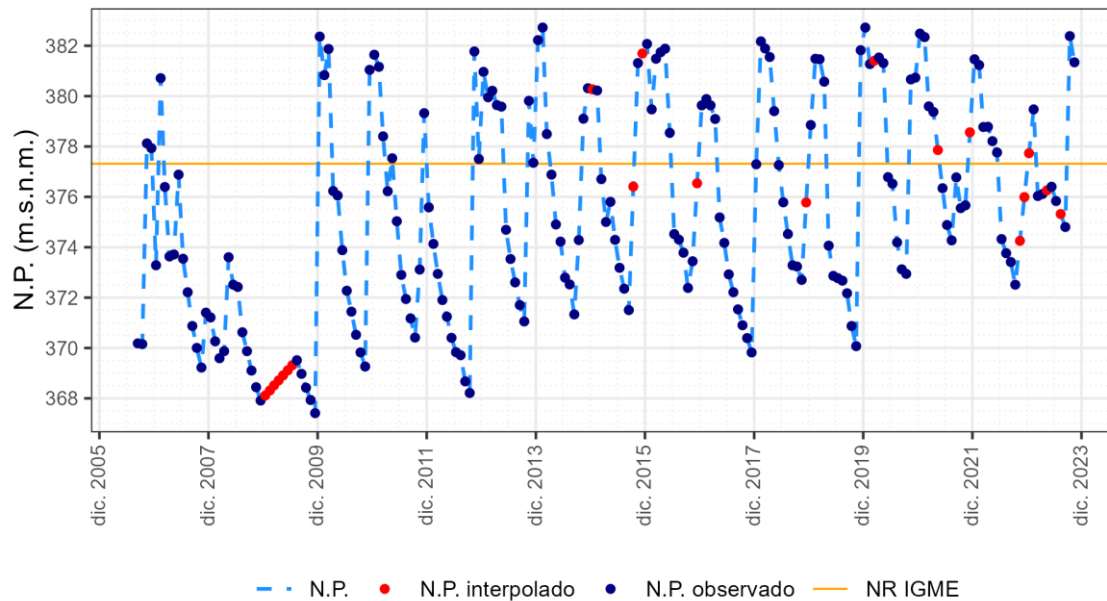
ES030MSBT030.023. Piez.: 03.10.001 - Torrejón el Rubio
