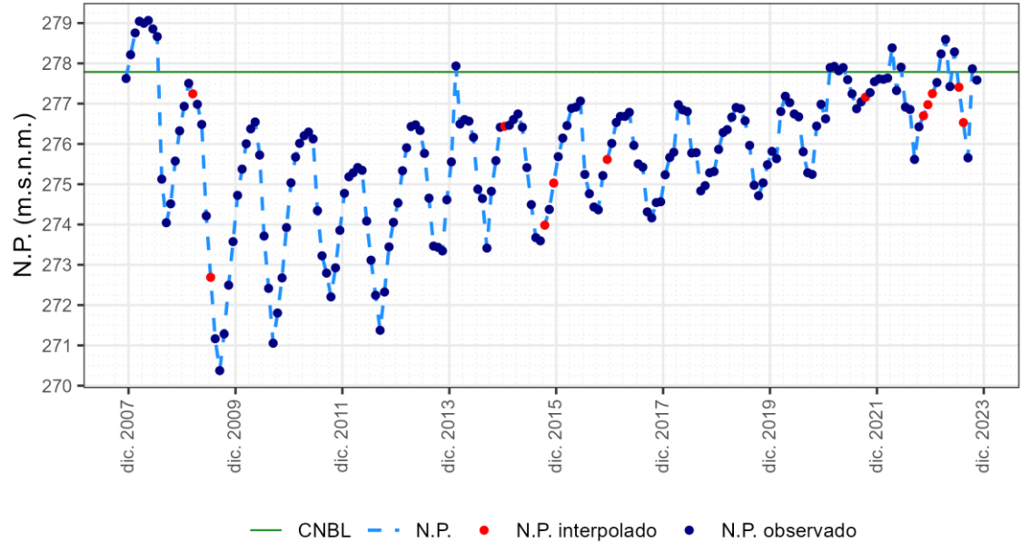
ES030MSBT030.022. Piez.: 03.09.005 - Pueblonuevo de Miramontes Cota superficie piezómetro = 289 msnm; CNBL = 278 msnm; Nivel de referencia = 293 msnm
