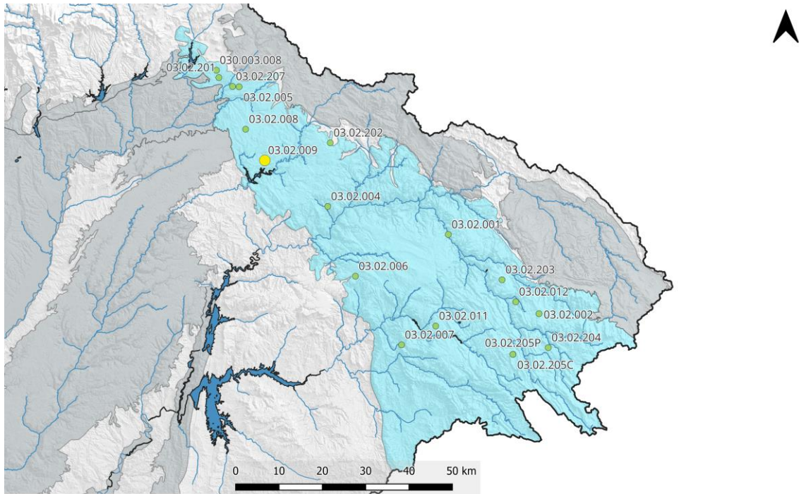
ES030MSBT030.003. Piez.: 03.02.009 - Torre Cuadrada de los Valles
