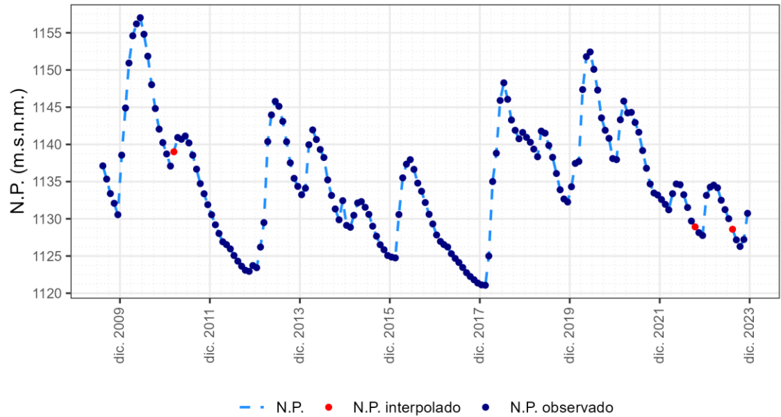
ES030MSBT030.002. Piez.: 03.99.203 - Torremocha del Pinar
