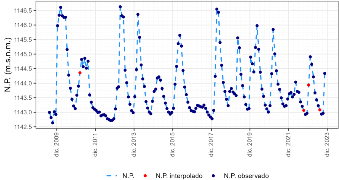
ES030MSBT030.003. Piez.: 03.02.202 - Sotodosos
