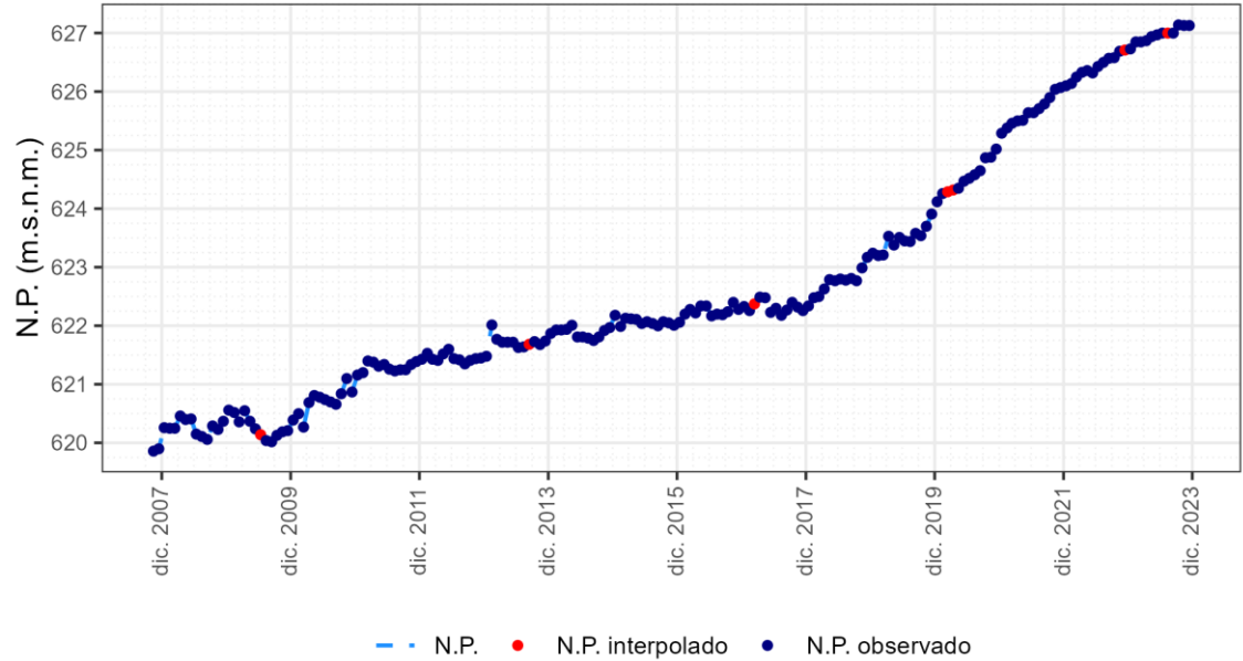
ES030MSBT030.011. Piez.: 03.05.049 - Parla
