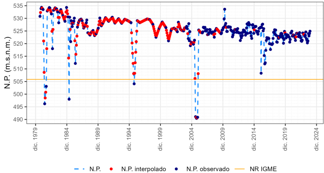
ES030MSBT030.015. Piez.: 03.05.073 - Olías del Rey
