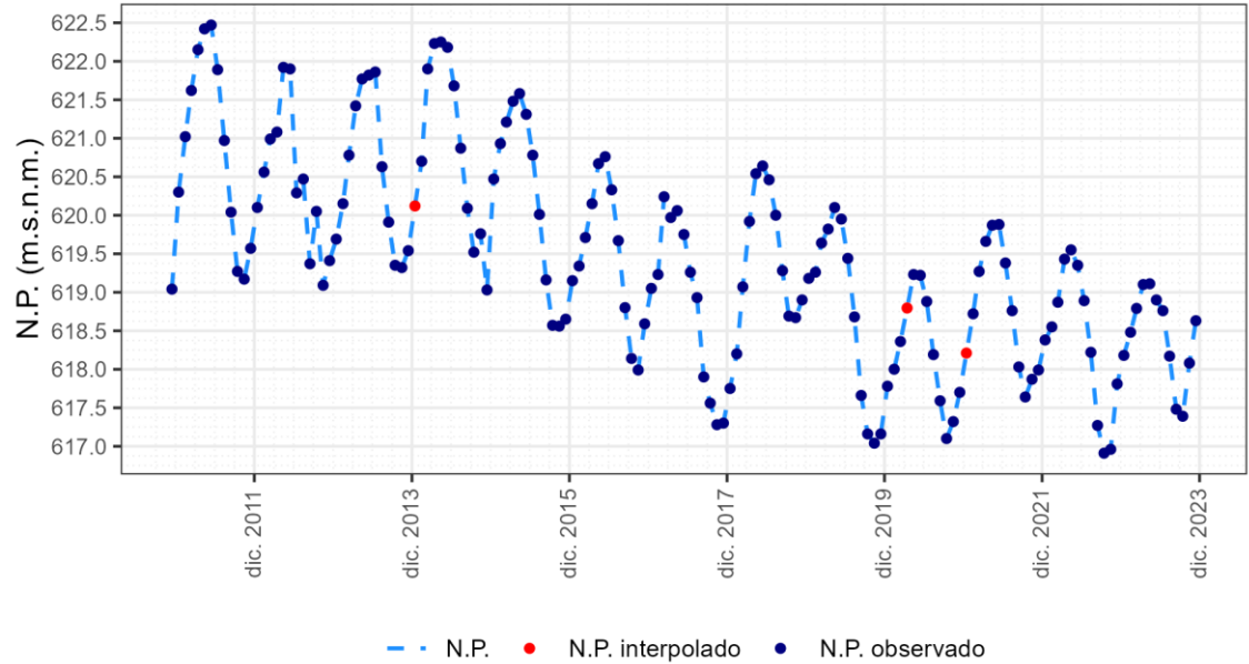
ES030MSBT030.010. Piez.: 03.03.012 - San Agustín de Guadalix
