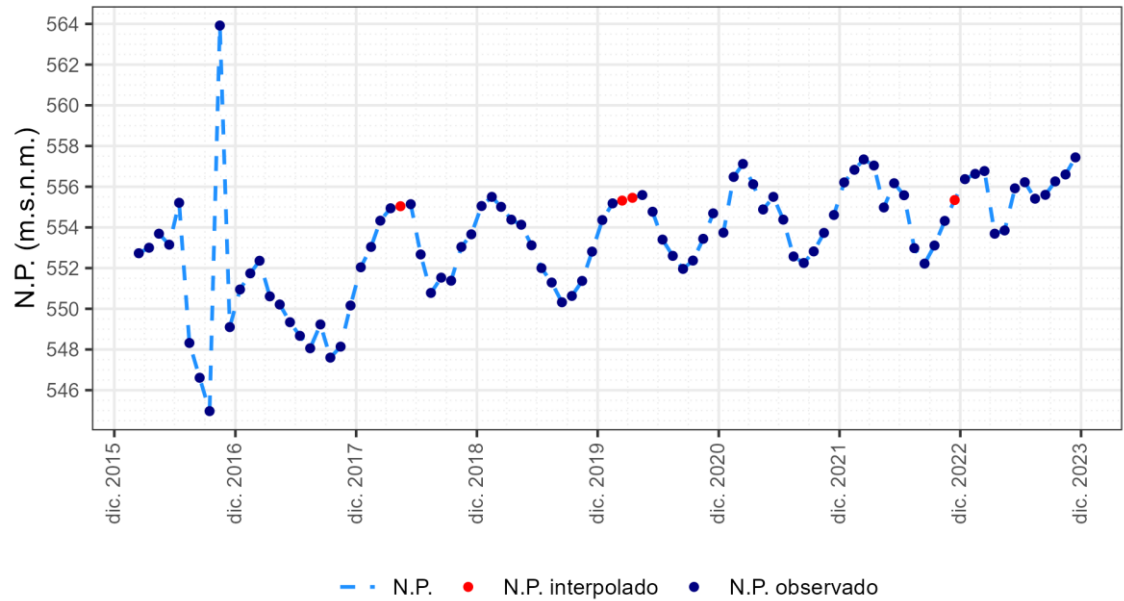
ES030MSBT030.012. Piez.: 030.012.001 - Villanueva de la Cañada
