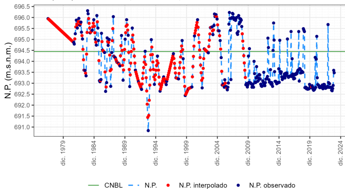
ES030MSBT030.004. Piez.: 03.03.007 - Patones
