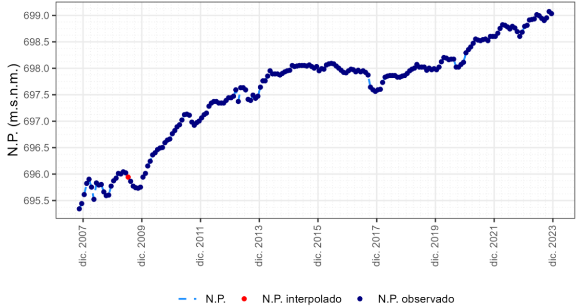
ES030MSBT030.006. Piez.: 03.04.005 - Cabanillas del Campo
