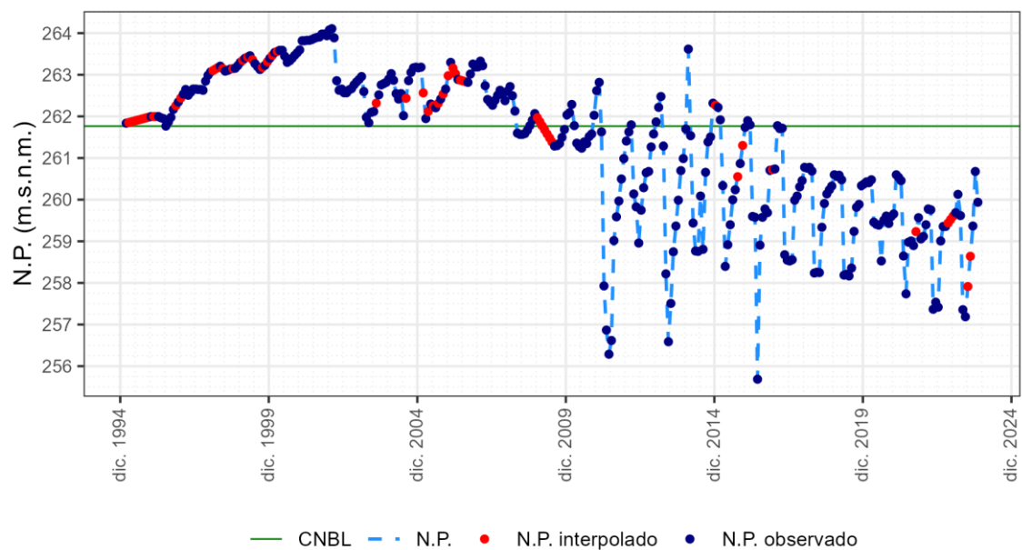
ES030MSBT030.022. Piez.: 03.09.011 - Rosalejo
