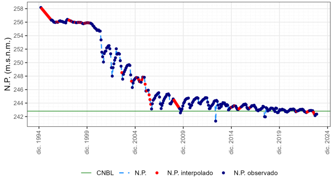
ES030MSBT030.022. Piez.: 03.09.012 - Talayueta
