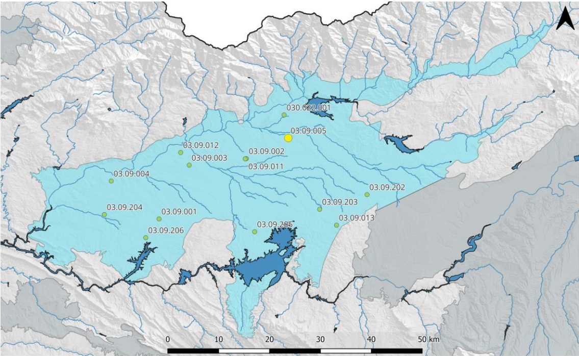
ES030MSBT030.022. Piez.: 03.09.005 - Pueblonuevo de Miramontes Cota superficie piezómetro = 289 msnm; CNBL = 278 msnm; Nivel de referencia = 293 msnm
