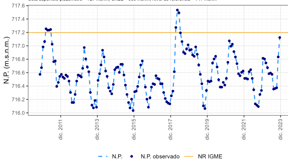
ES030MSBT030.006. Piez.: 03.04.025 - Yunque de Henares
