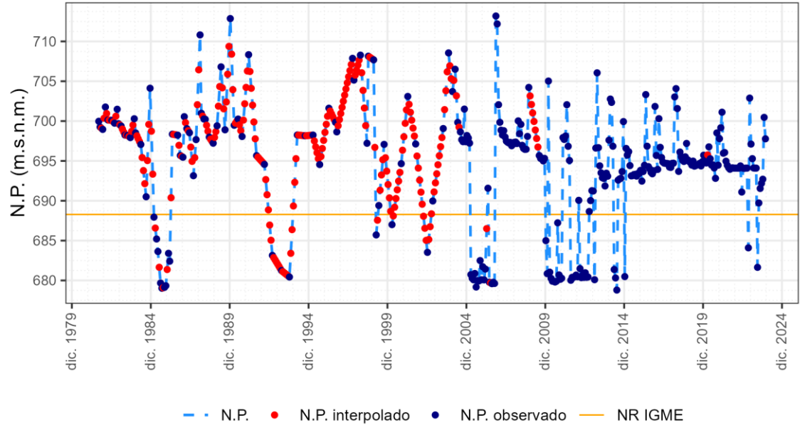
ES030MSBT030.004. Piez.: 03.03.005 - Torremocha del Jarama
