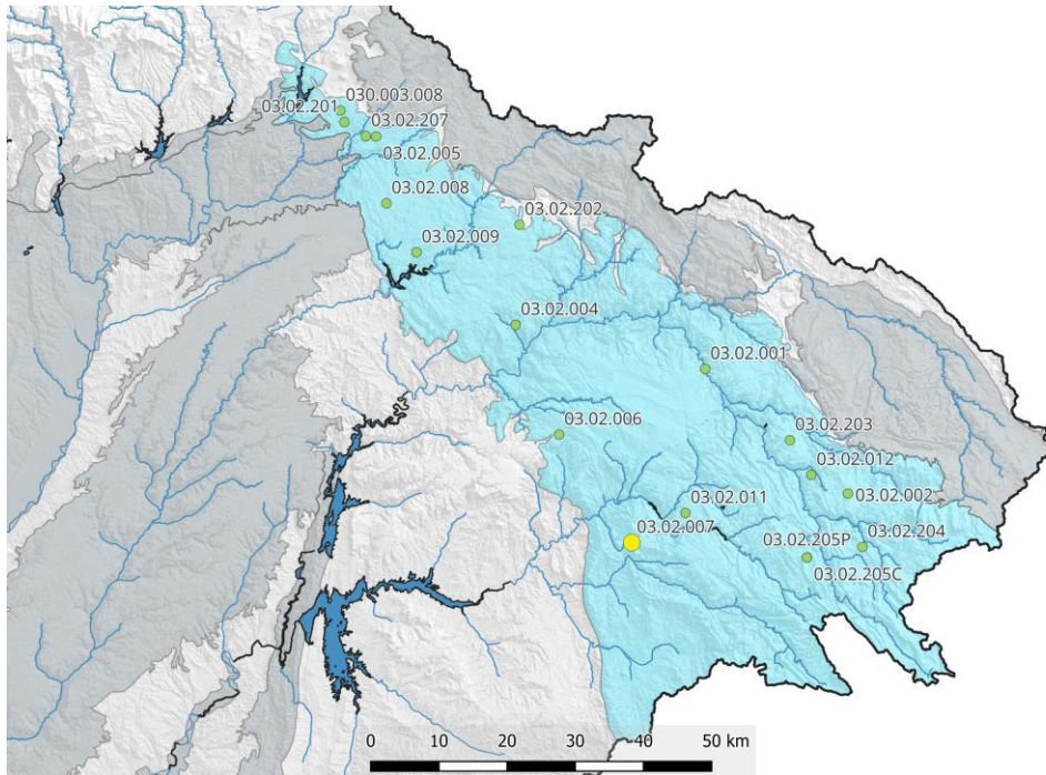
ES030MSBT030.003. Piez.: 03.02.007 - Cañizares
