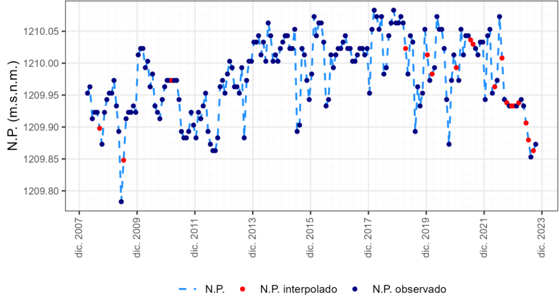
ES030MSBT030.003. Piez.: 03.02.012 - Peralejos de las Truchas Cota superficie piezómetro = 1392 msnm; CNBL = 1203 msnm; Nivel de referencia = 1276 msnm
