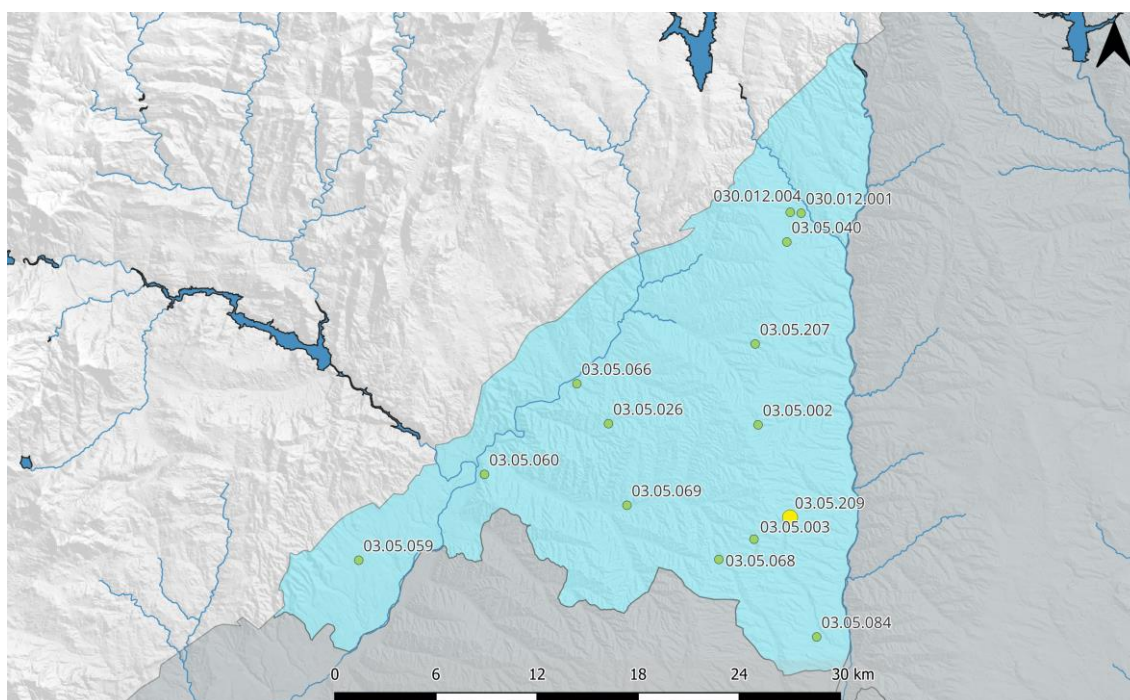
ES030MSBT030.012. Piez.: 03.05.209 - Navalcarnero
