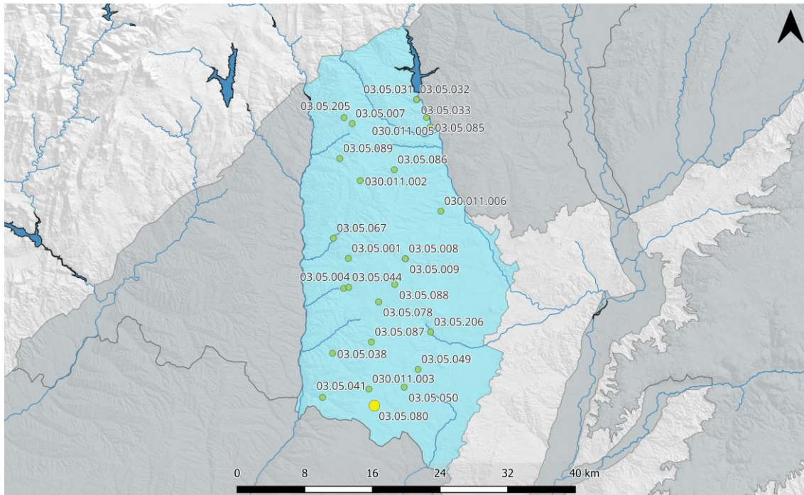
ES030MSBT030.011. Piez.: 03.05.080 - Grijón
