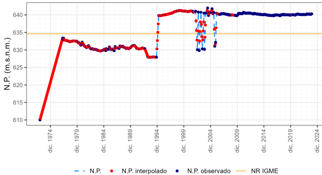
ES030MSBT030.011. Piez.: 03.05.080 - Grijón
