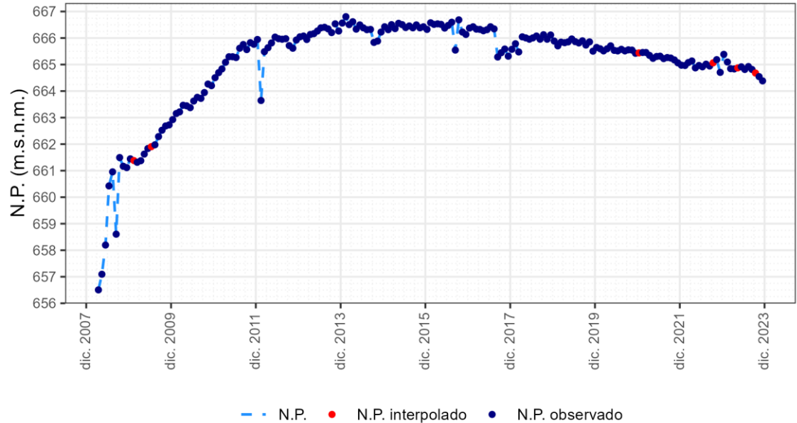
ES030MSBT030.014. Piez.: 03.07.001 - Almonacid de Zorita
