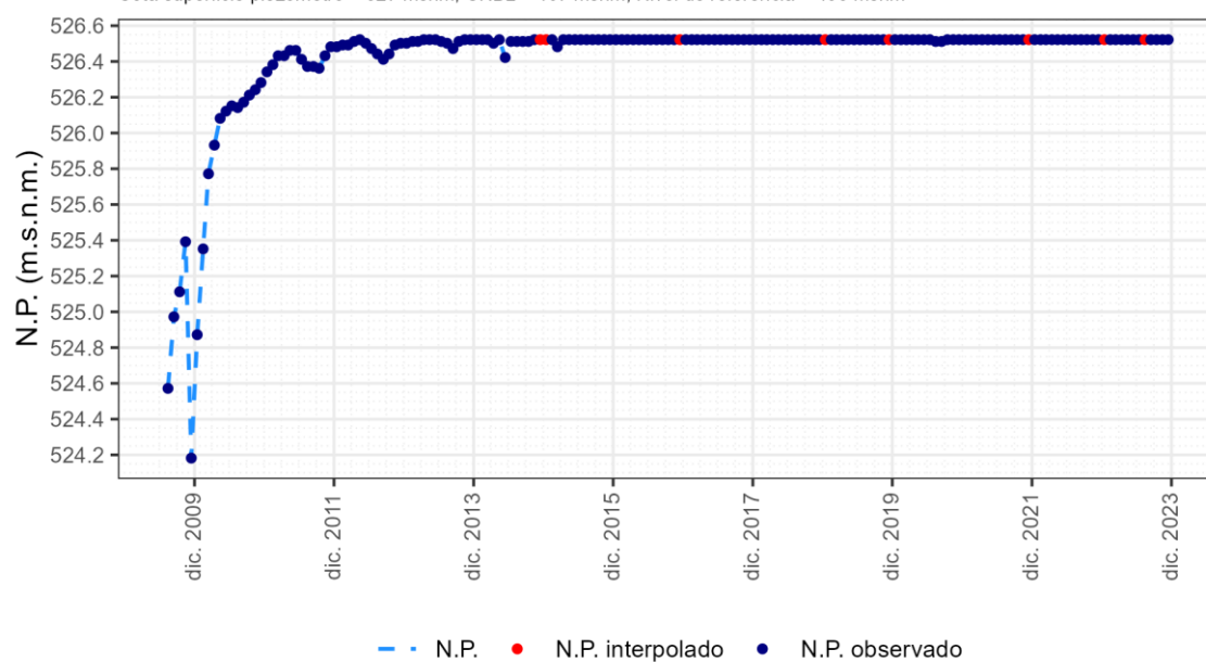
ES030MSBT030.015. Piez.: 03.05.202 - Numancia de la Sagra
