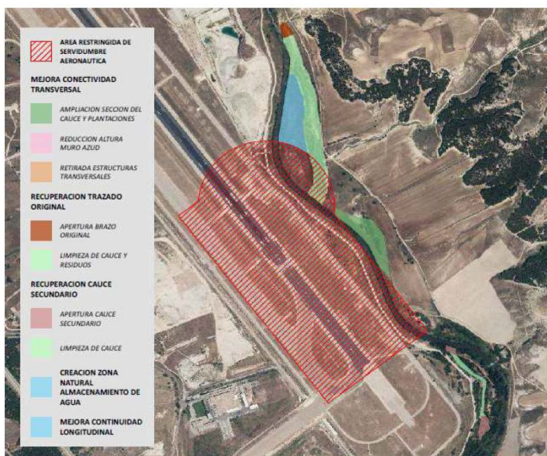
Figura 4.- Actuaciones planteadas en las inmediaciones del Aeropuerto
