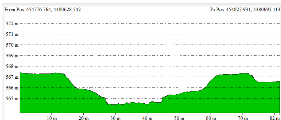
Figura 2.- Perfil transversal del tramo desviado
