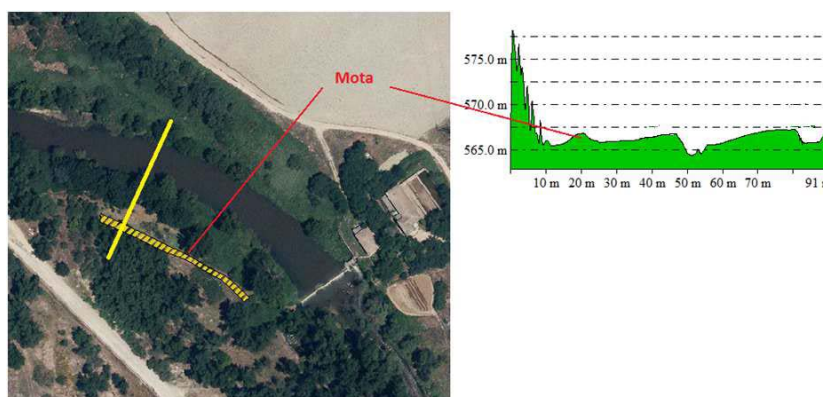
Figura 5.- Situación de la mota y perfil transversal
