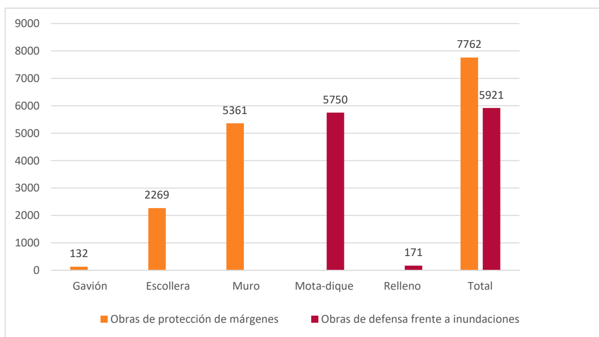
Figura 1.- Distribución de obras longitudinales de protección según funcionalidad y tipología.
