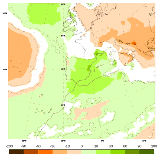
Anomalia de precipitación acumulada. Unidades: mm. Validez: del 9 de marzo de 2026 al 15 de marzo de 2026.
