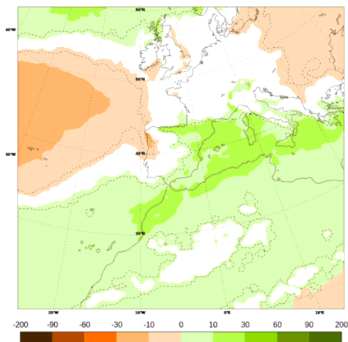
Anomalia de precipitación acumulada. Unidades: mm. Validez: del 16 de marzo de 2026 al 22 de marzo de 2026.
