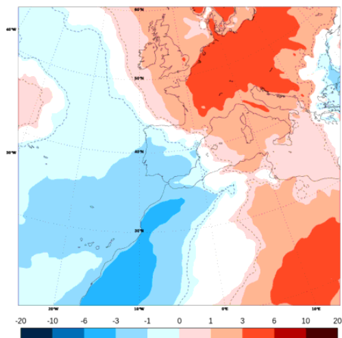
Anomalia de temperatura a 2 m. Unidades: °C. Validez: del 9 de marzo de 2026 al 15 de marzo de 2026.
