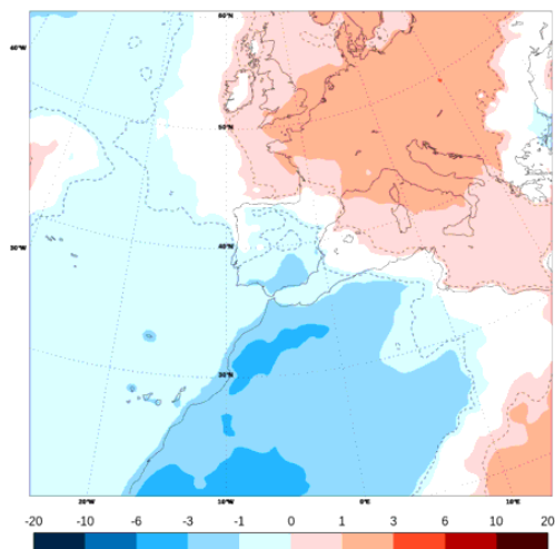
Anomalia de temperatura a 2 m. Unidades: °C. Validez: del 16 de marzo de 2026 al 22 de marzo de 2026.
