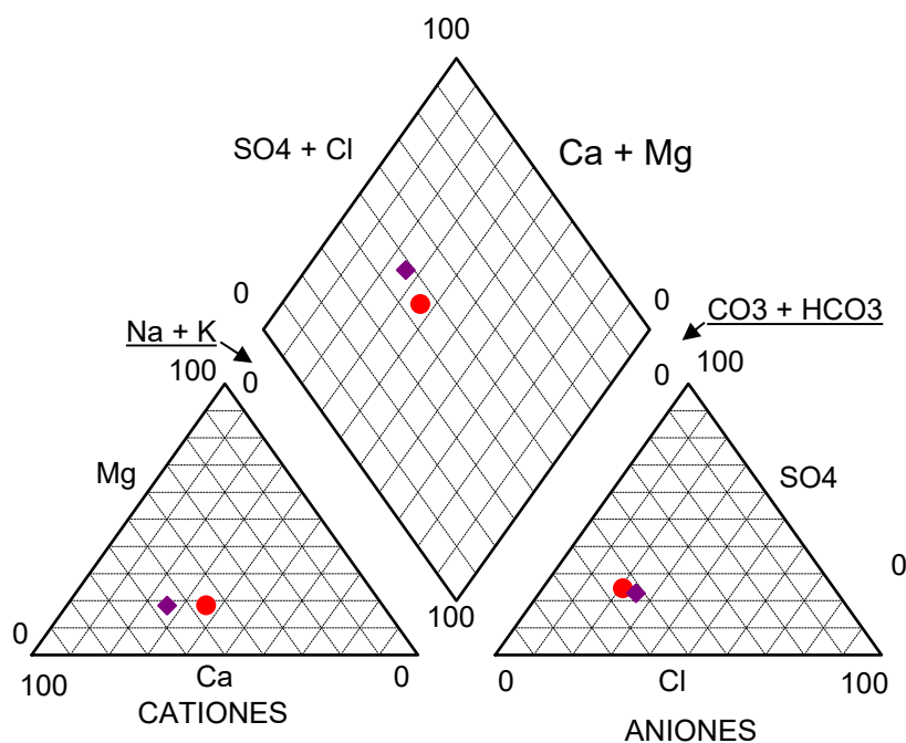
DIAGRAMA DE PIPER DE LAS ESTACIONES DE CONTROL DE LA MASA DE AGUA 030.020
