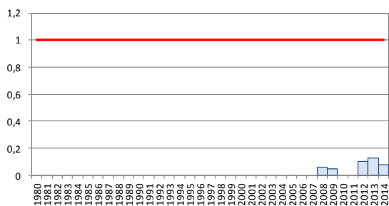
ES030MSPF0912010. Est: TA62210003. Amonio. Media anual
