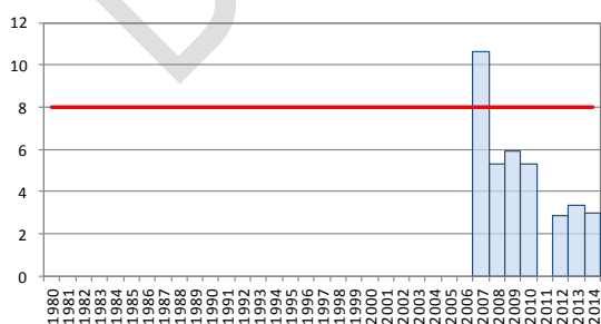
ES030MSPF0403010. Est: TA53306007. DBO5. Media anual
