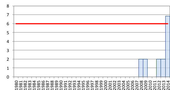
ES030MSPF0912010. Est: TA62210003. DBO5. Media anual
