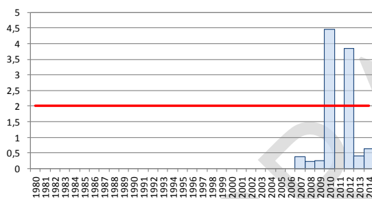
ES030MSPF0409021. Est: TA55806001. Amonio. Media anual
