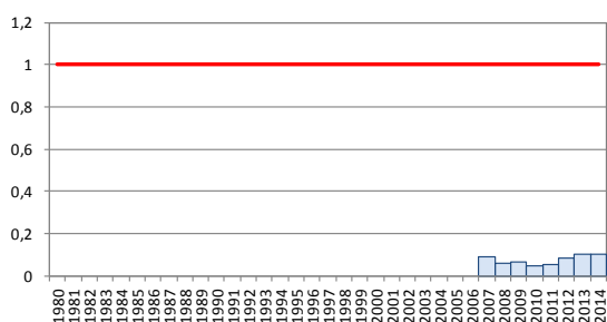
ES030MSPF0614010. Est: TA62708007. Amonio. Media anual
