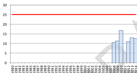
ES030MSPF0118010. Est: TA56102001. Nitratos. Media anual
