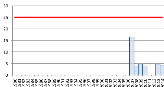
ES030MSPF0517010. Est: TA58007014. Nitratos. Media anual
