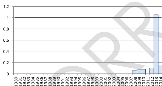
ES030MSPF0519010. Est: TA55807001. Amonio. Media anual
