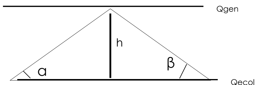
Figura 10. Volumen del caudal generador; Tasa de cambio subida = Tangente \alpha ; Tasa de cambio bajada = Tangente \beta ; h = \text{MCO} - \text{Q ecol}
