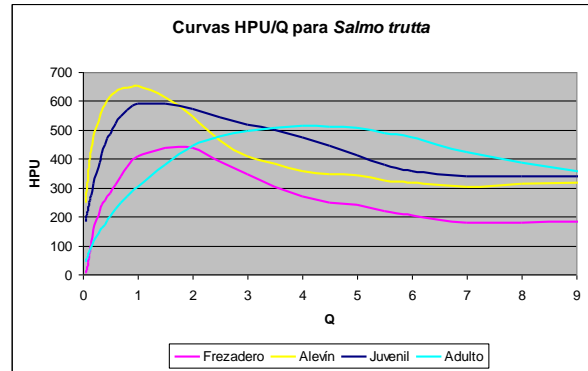
Figura 6. Ejemplo Curvas HPU/Q para otro cauce modelo
