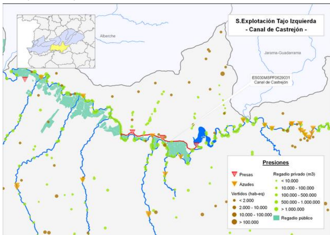
Figura 49. Principales presiones sobre el Canal de Castrejón
