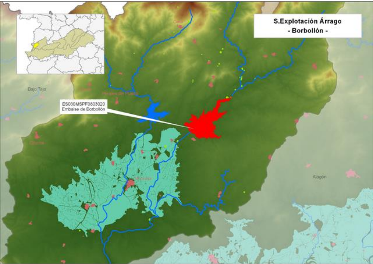
Figura 64. Agrupación de masas de agua del SE Árrago: Borbollón
