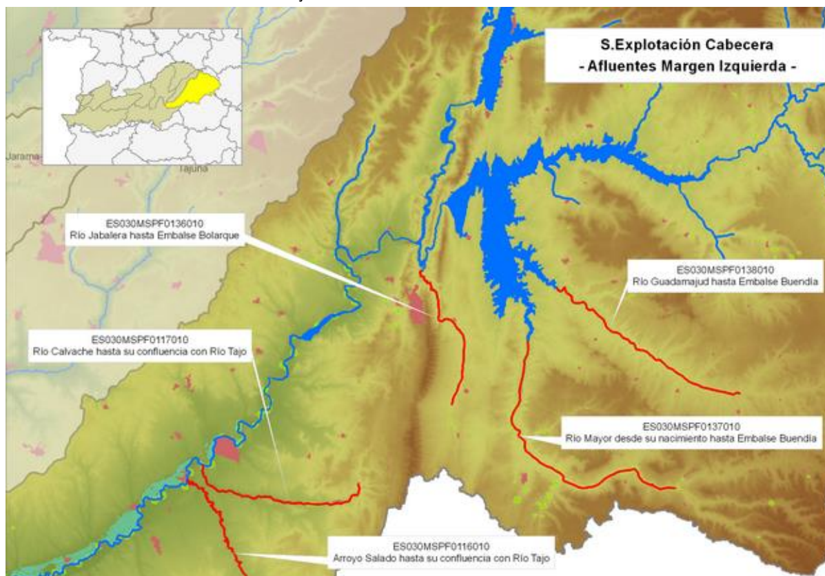
Figura 7. Agrupación de masas del SE Cabecera: Afluentes de la margen izquierda del río Tajo
