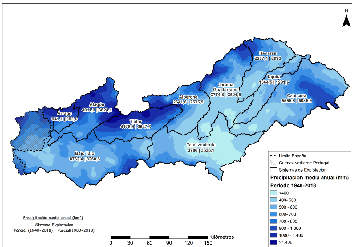
Figura 5. Precipitación media anual por sistema de explotación parcial, en hm³/año, según el modelo SIMPA.
