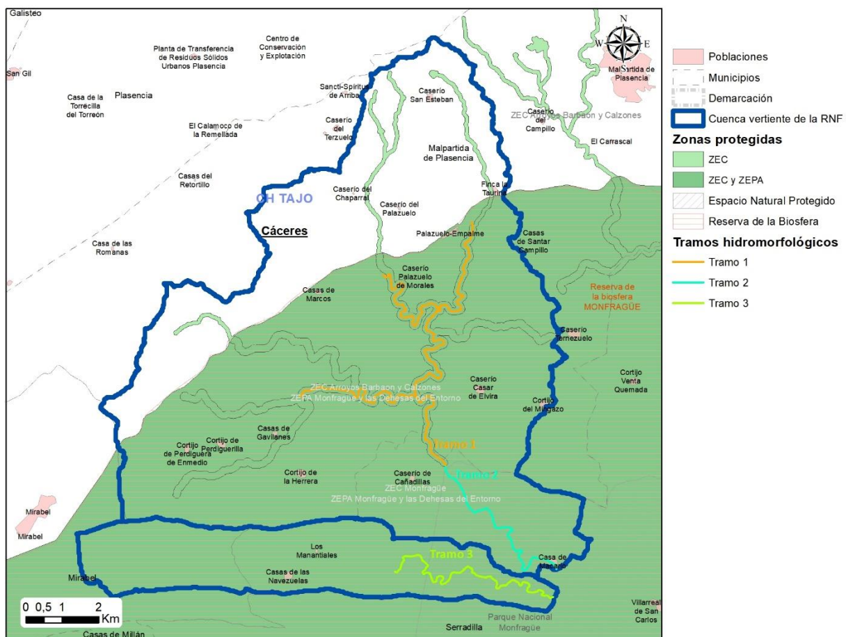
Tramos hidromorfológicos de la Reserva Natural Fluvial Río Barbaón
