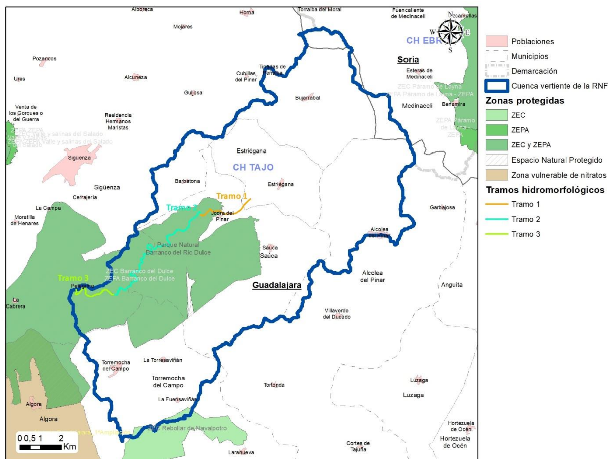
Tramos hidromorfológicos de la Reserva Natural Fluvial Río Dulce
