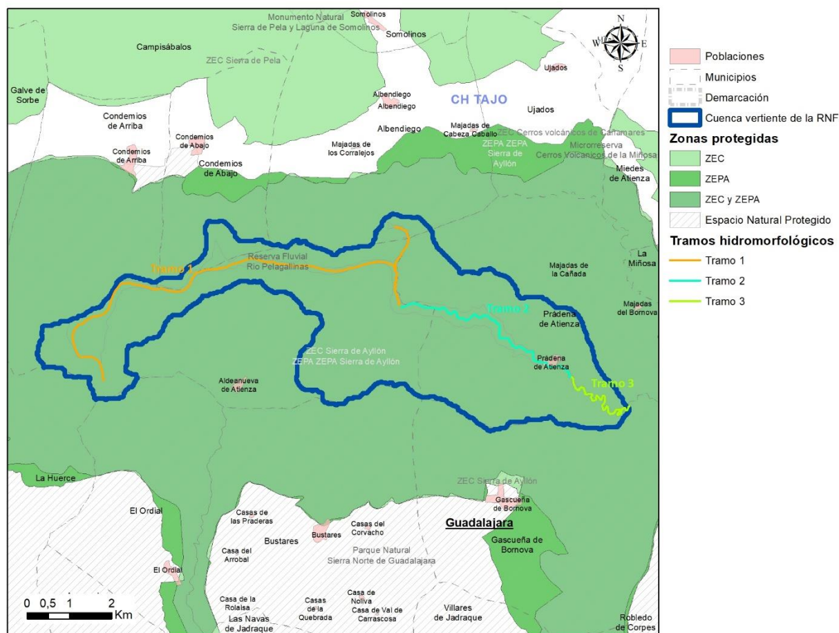
Tramos hidromorfológicos de la Reserva Natural Fluvial Río Pelagallinas
