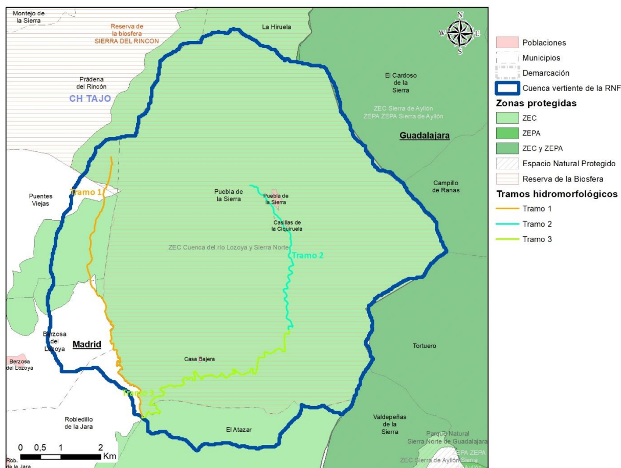
Tramos hidromorfológicos de la Reserva Natural Fluvial Ríos Riato y Puebla
