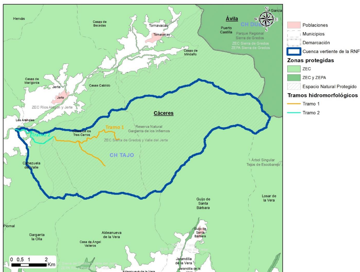
Tramos hidromorfológicos de la Reserva Natural Fluvial Garganta de los Infiernos
