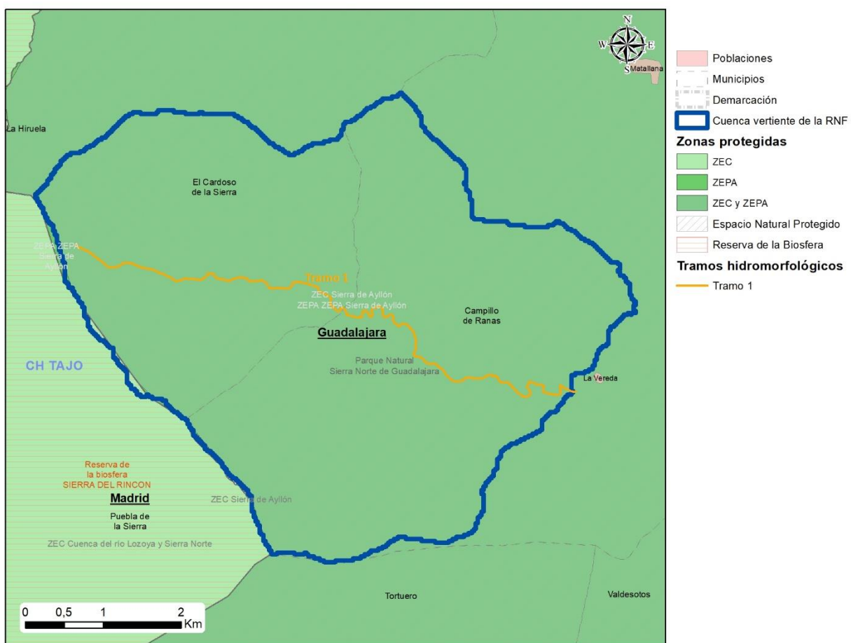
Tramos hidromorfológicos de la Reserva Natural Fluvial Arroyo Vallosera
