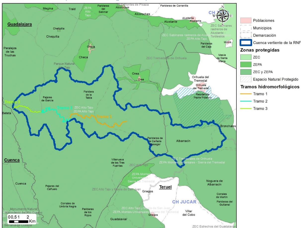
Tramos hidromorfológicos de la Reserva Natural Fluvial Río Hozseca
