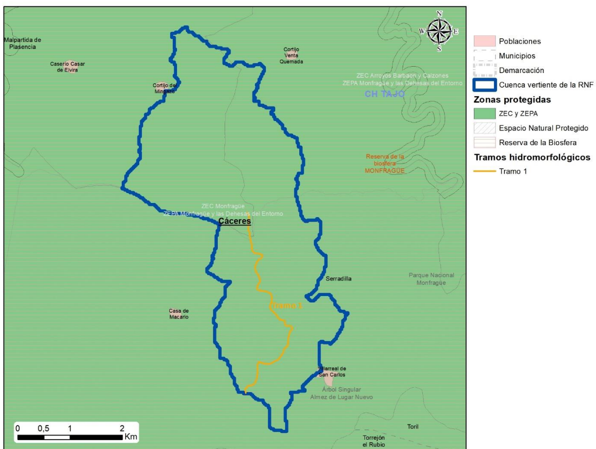
Tramos hidromorfológicos de la Reserva Natural Fluvial Río Malvecino
