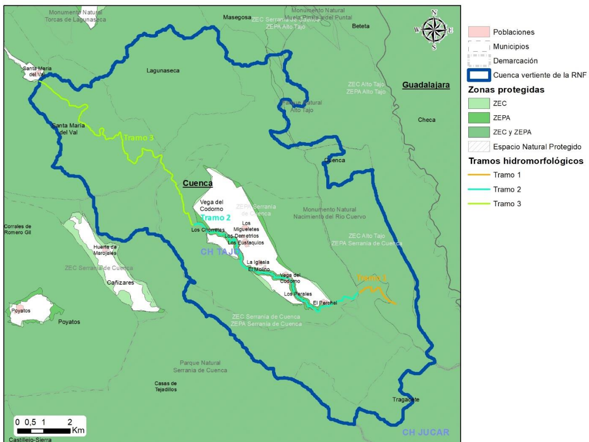
Tramos hidromorfológicos de la Reserva Natural Fluvial Río Cuervo
