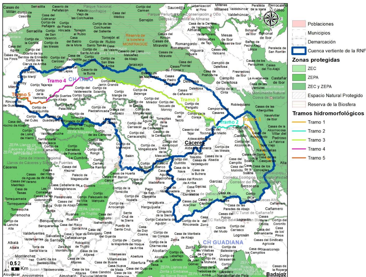
Tramos hidromorfológicos de la Reserva Natural Fluvial Río Almonte
