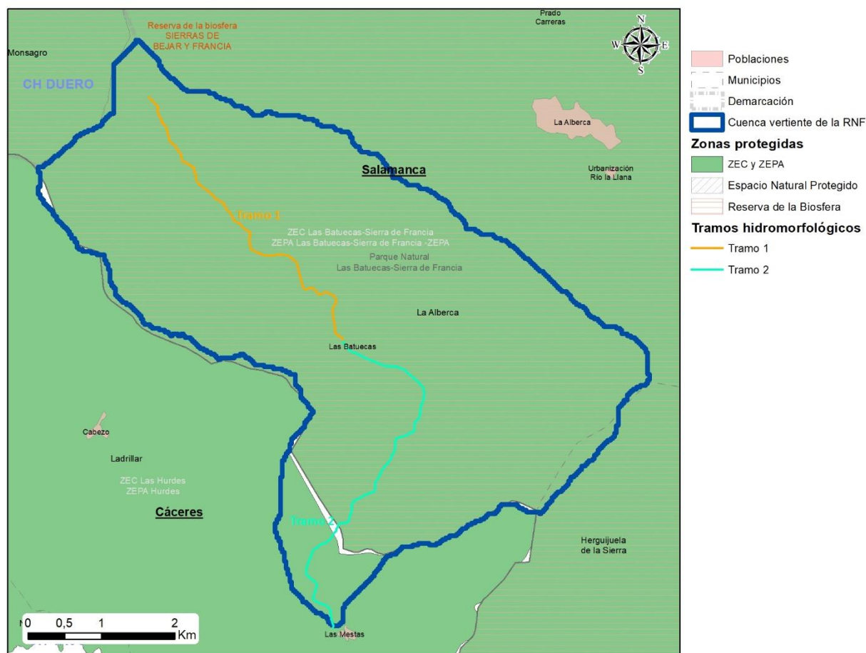
Tramos hidromorfológicos de la Reserva Natural Fluvial Río Batuecas
