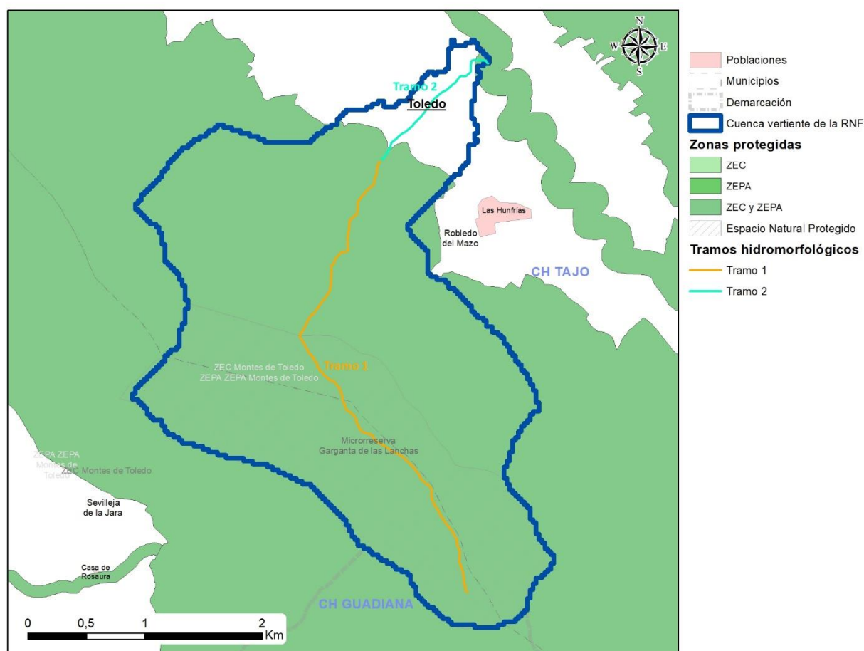
Tramos hidromorfológicos de la Reserva Natural Fluvial Garganta de las Lanchas
