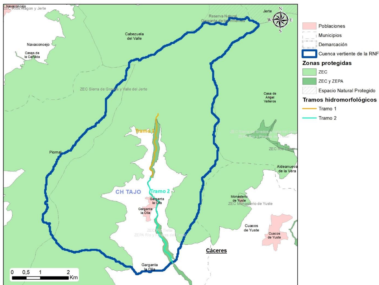
Tramos hidromorfológicos de la Reserva Natural Fluvial Garganta Mayor
