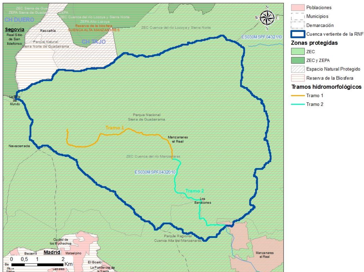
Tramos hidromorfológicos de la Reserva Natural Fluvial del río Manzanares
