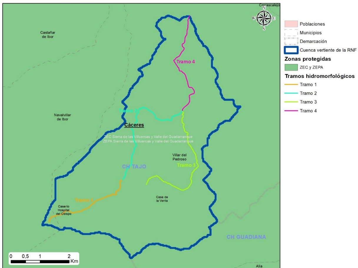
Tramos hidromorfológicos de la Reserva Natural Fluvial Río Mesto
