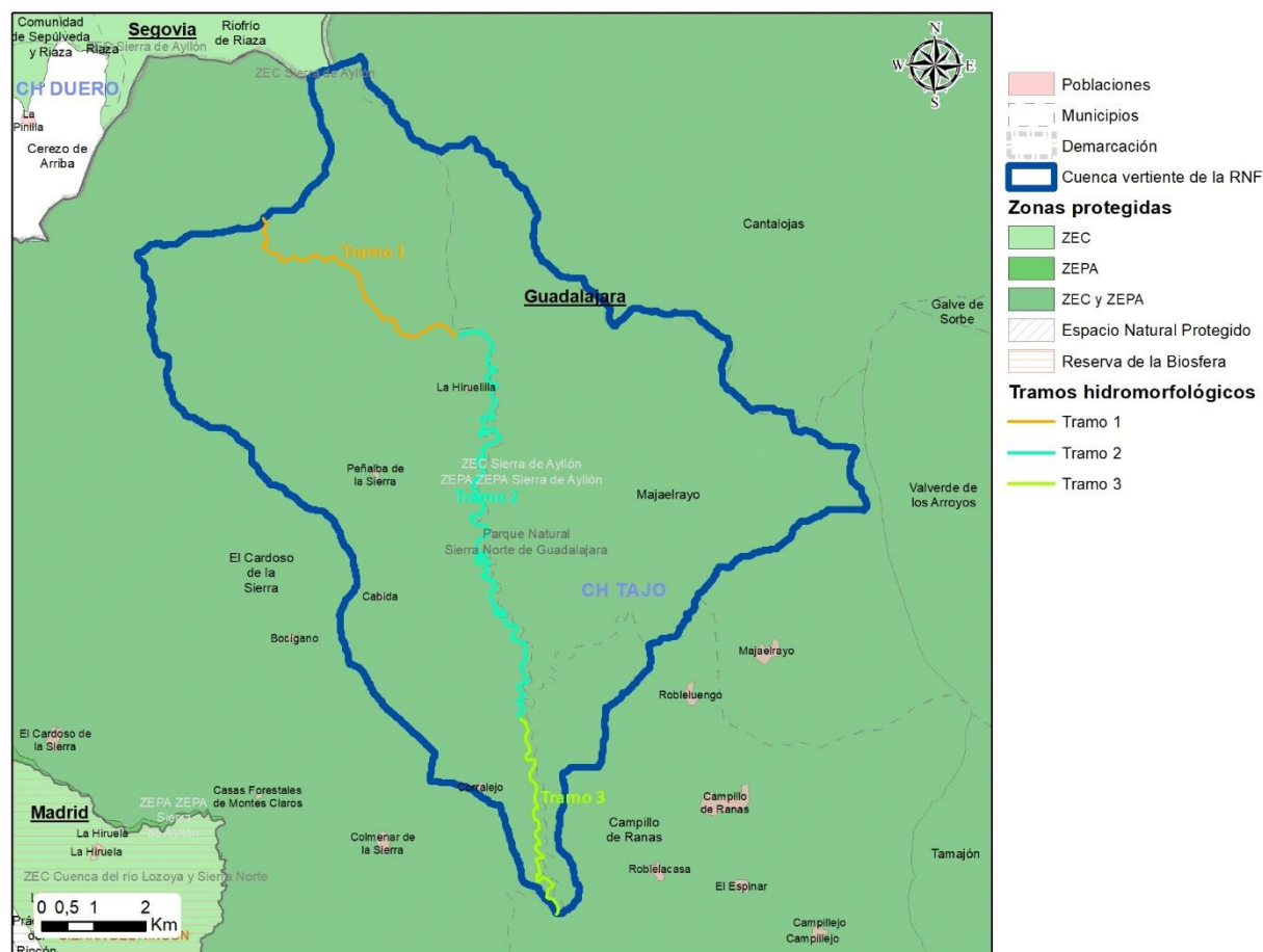
Tramos hidromorfológicos de la Reserva Natural Fluvial Río Jaramilla
