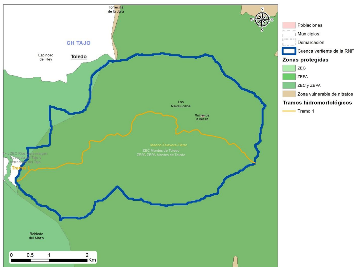
Tramos hidromorfológicos de la Reserva Natural Fluvial Arroyo Cabrera
