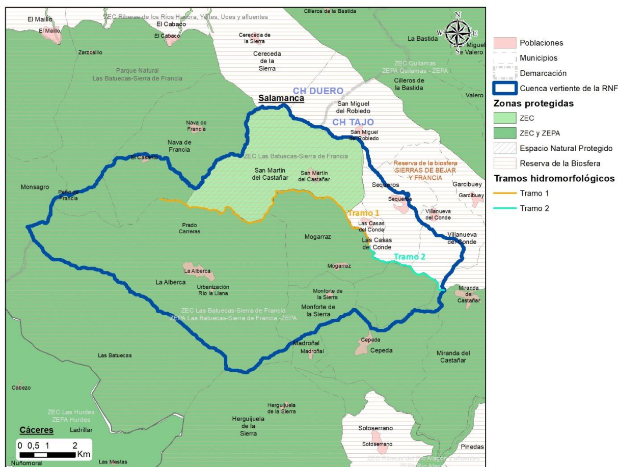
Tramos hidromorfológicos de la Reserva Natural Fluvial Río Francia
