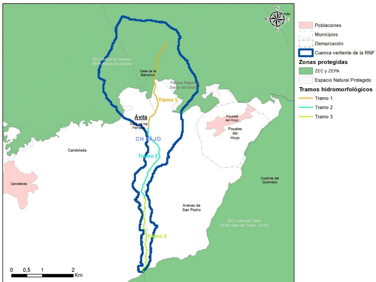
Tramos hidromorfológicos de la Reserva Natural Fluvial Río Muelas
