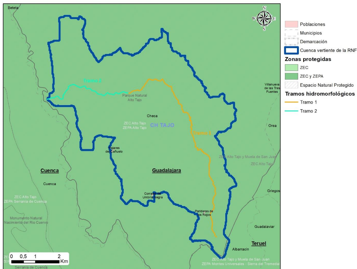
Tramos hidromorfológicos de la Reserva Natural Fluvial Arroyo los Huecos
