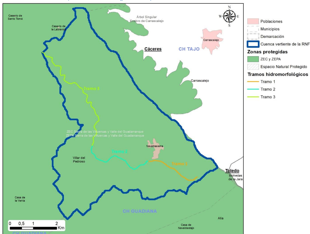
Tramos hidromorfológicos de la Reserva Natural Fluvial Río Gualija
