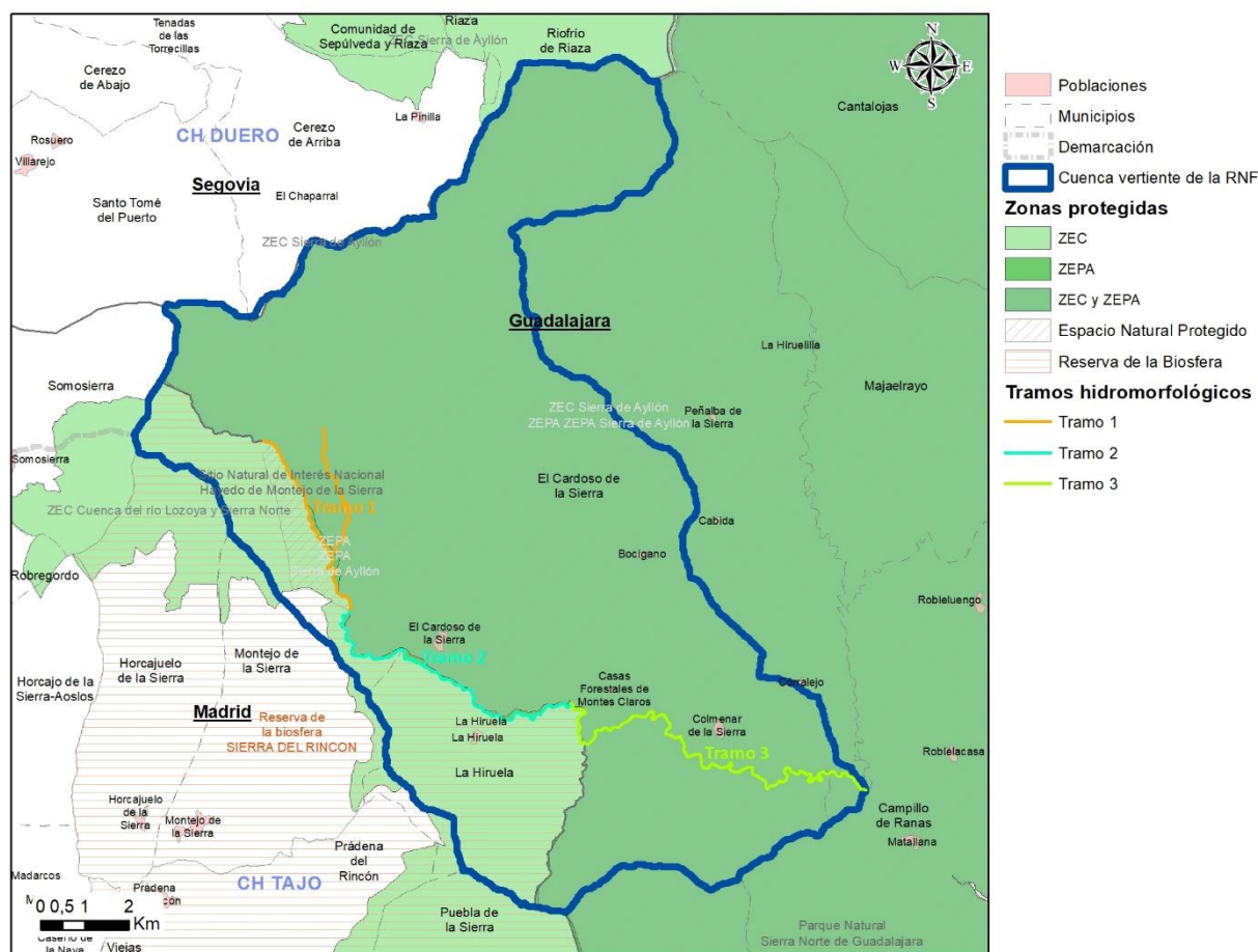
Tramos hidromorfológicos de la Reserva Natural Fluvial Río Jarama
