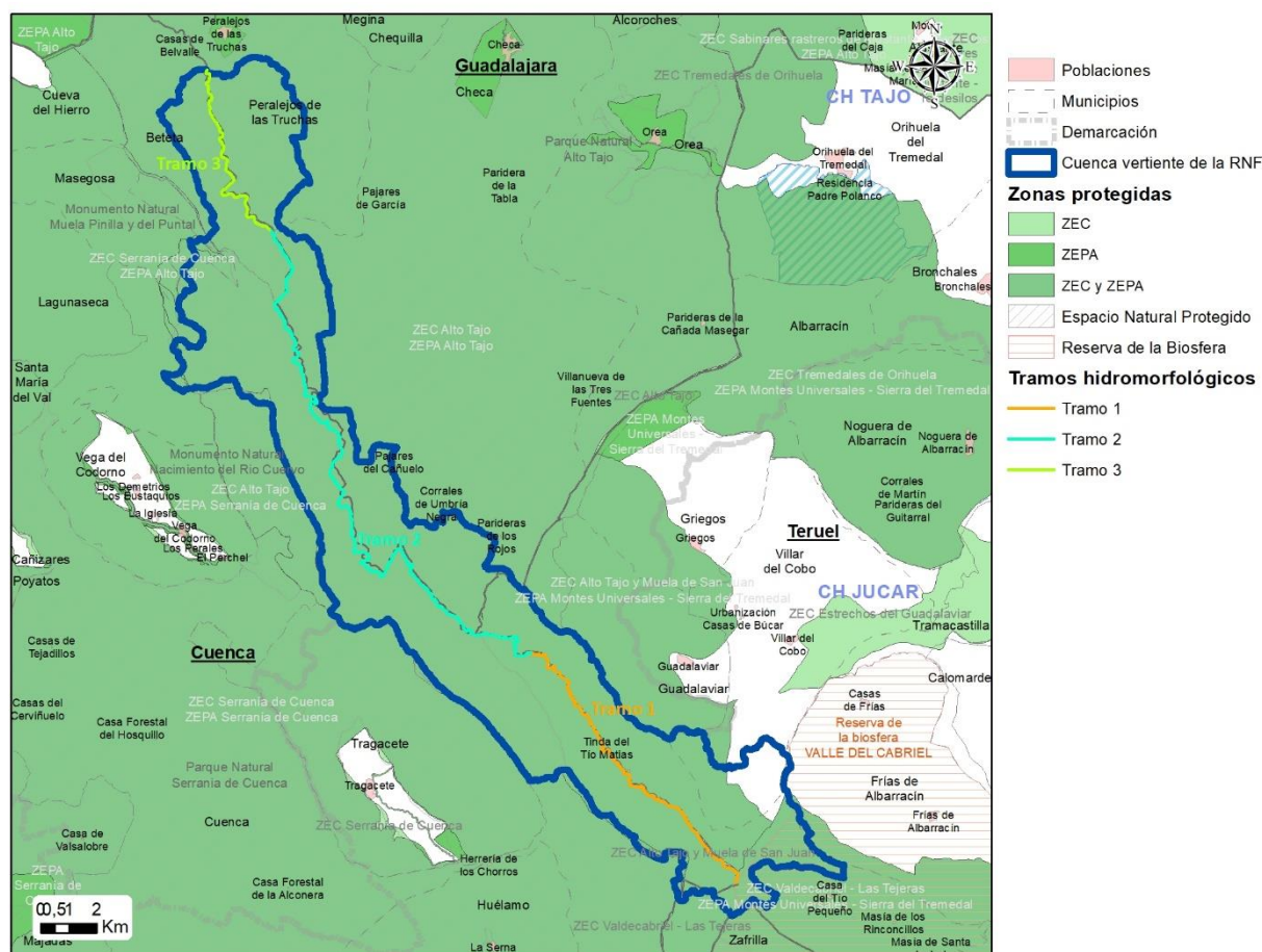
Tramos hidromorfológicos de la Reserva Natural Fluvial Río Tajo
