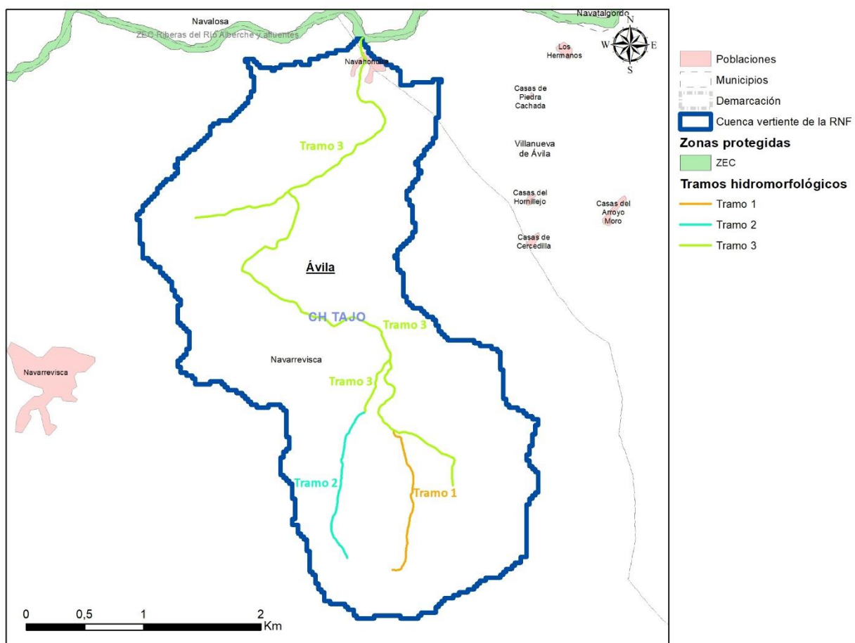
Tramos hidromorfológicos de la Reserva Natural Fluvial Río Navahondilla
