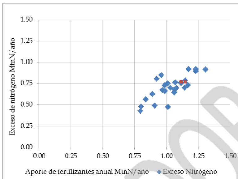
Figura 19. Relación entre el aporte de fertilizantes y el exceso anual de nitrógeno (Millones de tnN/año).
