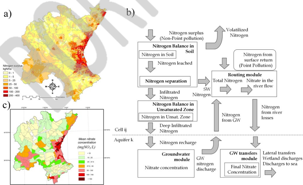
Figura 13. Modelo de simulación de nitrato Patrical (Perez-Martin, 2016).
