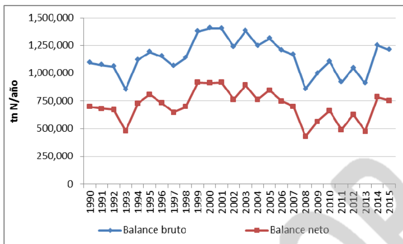
Figura 6. Balance bruto y balance neto de nitrógeno en la agricultura Española, periodo 1990-2015.
