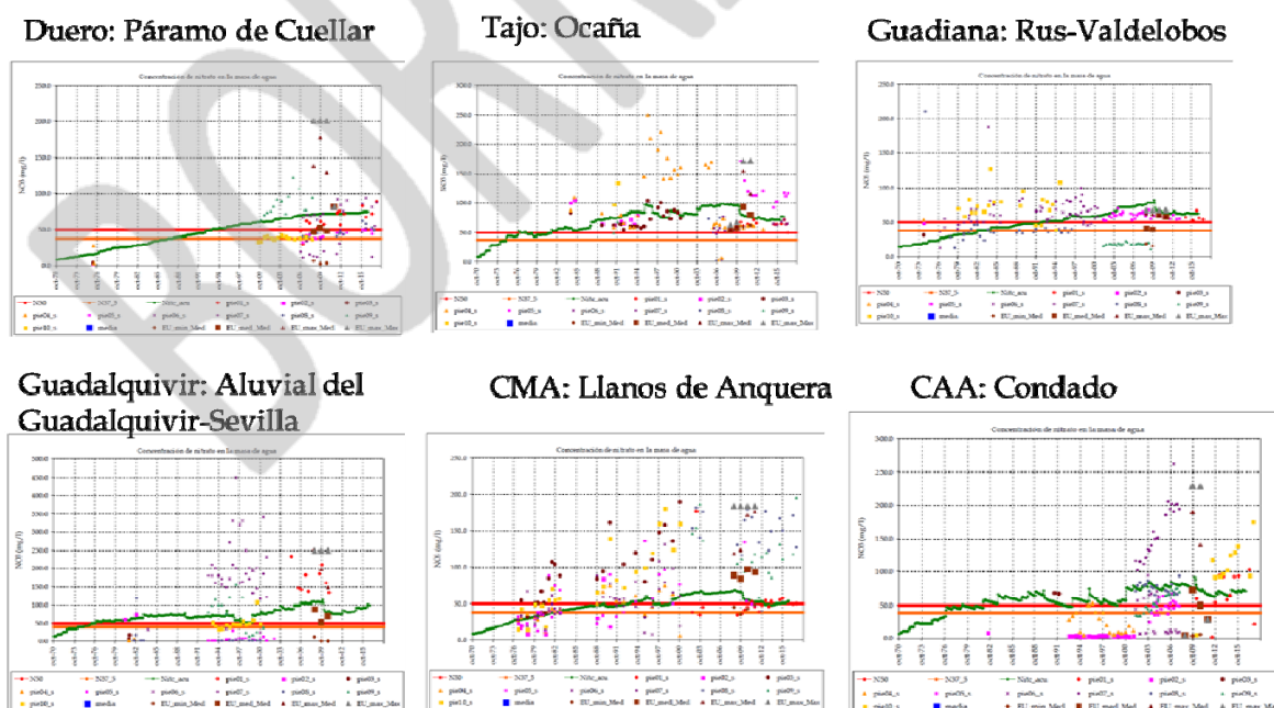
Figura 14. Gráficos de calibración de la concentración de nitrato en sectores de masas de agua subterráneas.
