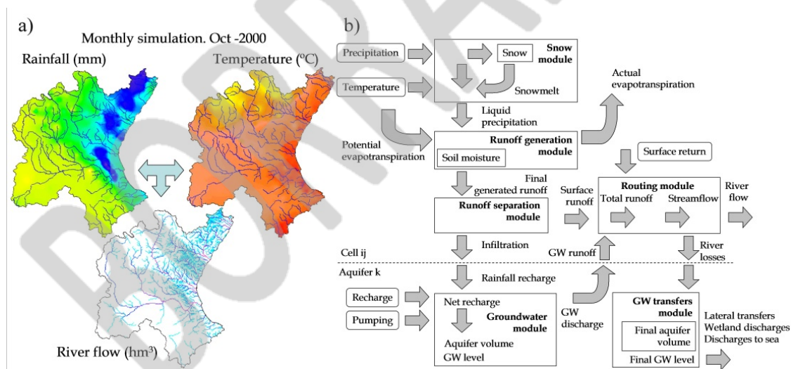
Figura 10. Precipitación, temperatura y aportación en la red fluvial en octubre de 2000 y esquema de funcionamiento del modelo Patrical (Perez-Martin et al., 2014).
