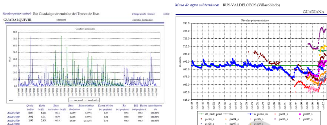
Figura 12. Caudales mensuales en régimen natural al embalse del Tranco de Beas en el río Guadalquivir (m³/s), y niveles piezométricos en la masa de agua subterráneas de Rus-Valdelobos (m.s.n.m.). Contraste entre el modelo y los datos históricos.
