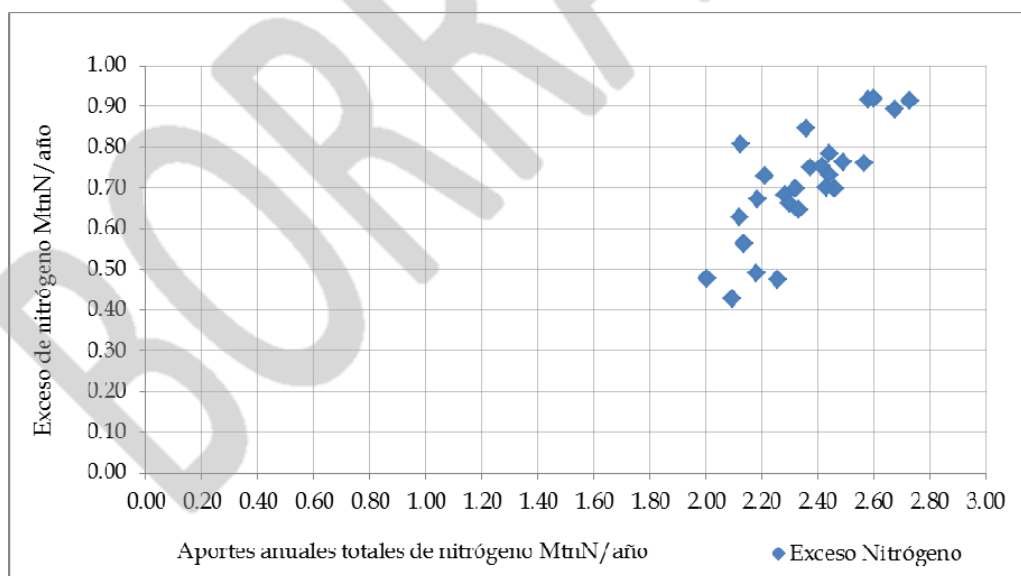
Figura 18. Relación entre el aporte total de nitrógeno y el exceso anual de nitrógeno (Millones de tnN/año).
