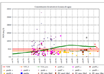
Figura 15. Gráficos de calibración de la concentración de nitrato en sectores de masas de agua subterráneas.
