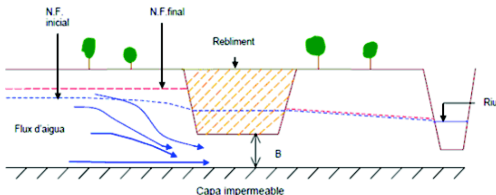
Il·lustració 51: Esquema de la modificació del nivel freático y del flujo del agua debido al relleno. Estudi Recomendacions per a la protecció de les aigües subterrànies front graveres. Dr. Ing. Jesús Carrera Otger Ferrer
