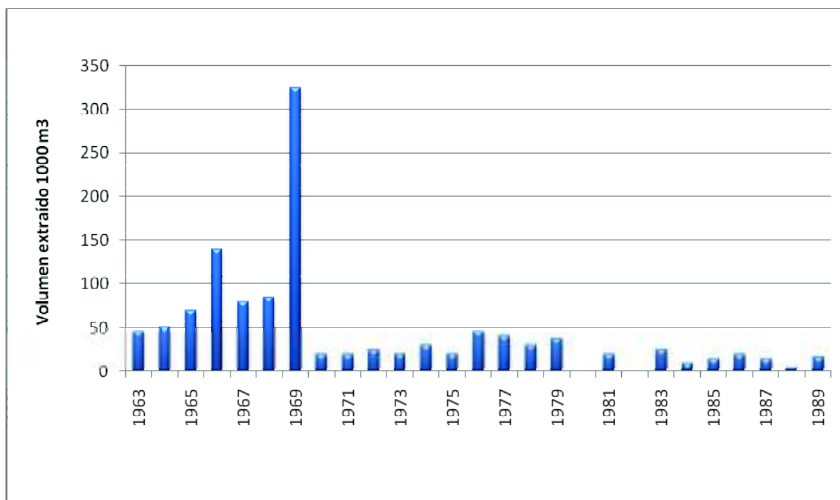
Ilustración 25: Evolución de la extracción de áridos en el río Gállego. Fuente: Estudio hidráulico y morfodinámico del río Gállego en Zaragoza.UPC. Dpto. de Ingeniería Hidráulica, M. Y A. Barcelona, junio de 2005
